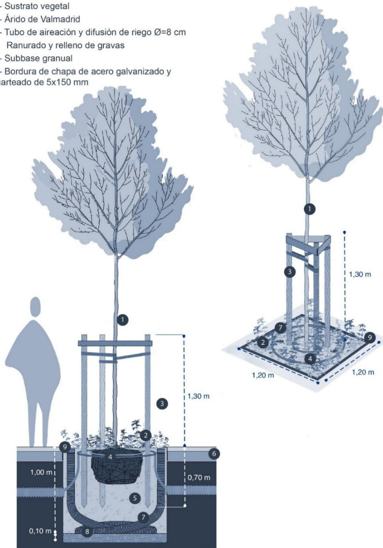
Imagen 21: Detalle de plantación en terrizo.
