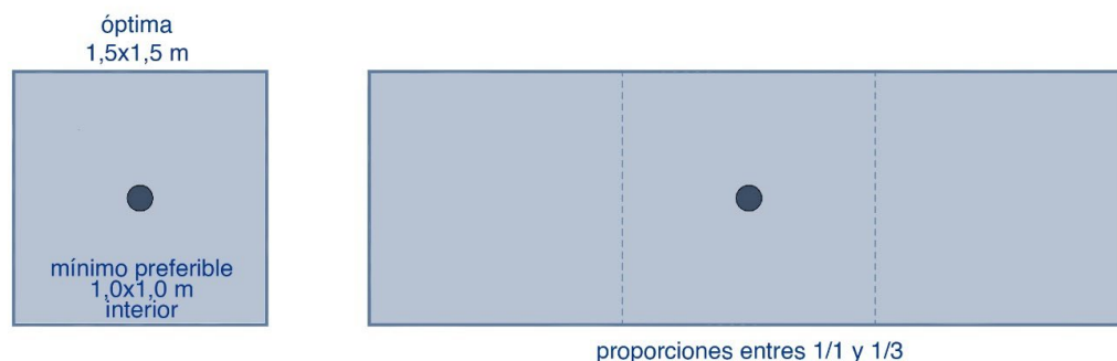
Imagen 24: Dimensiones de alcorques (medidas del interior).
