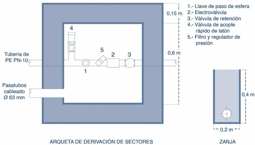
ARQUETA DE DERIVACIÓN DE SECTORES
