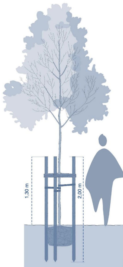
Imagen 15: Colocación de tutores de arbolado.
