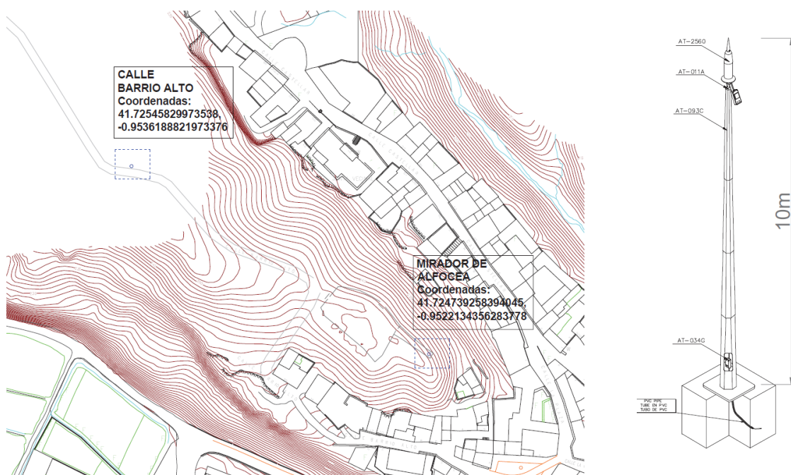
Figura 1. Localización de los emplazamientos y modelo del pararrayos
