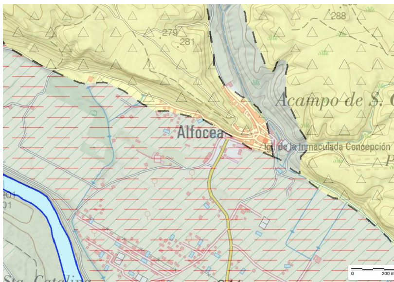
Figura 2. Situación geológica. Color amarillo: sustrato Terciario; color gris con tramas: recubrimiento Cuaternario.
