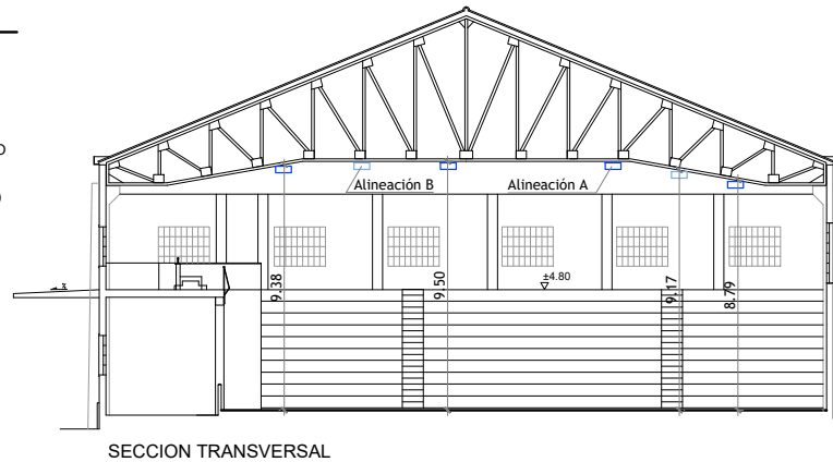
SECCION TRANSVERSAL
