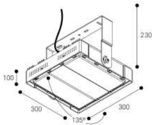
Dimensiones (mm):
