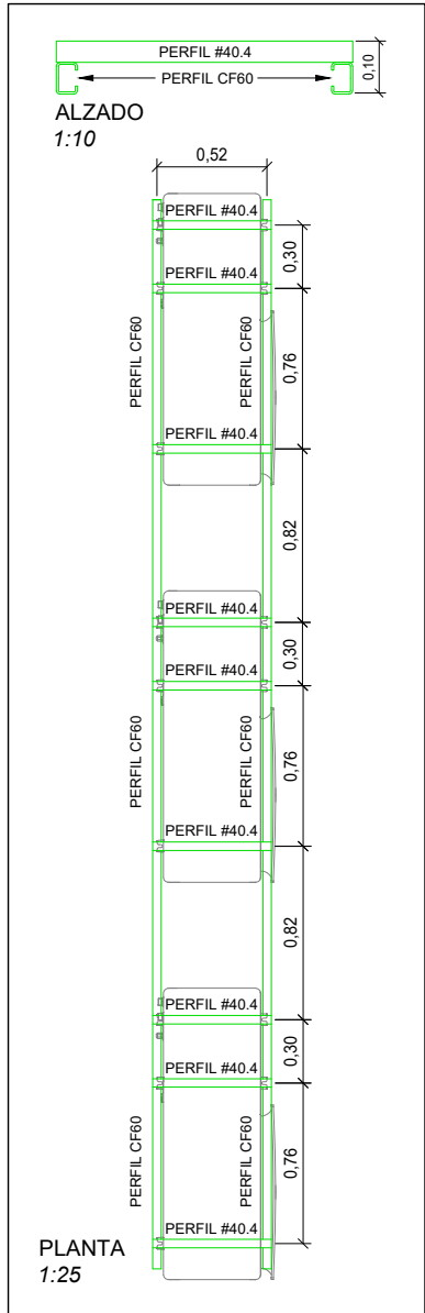
DETALLE BANCADA
