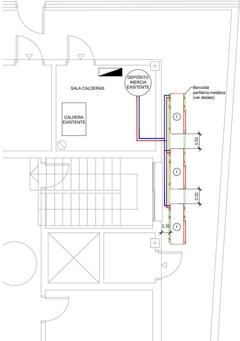
PLANTA 1:50
