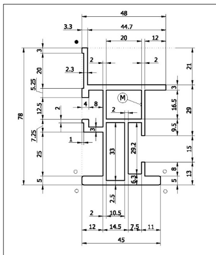
Sección marco aluminio módulos
