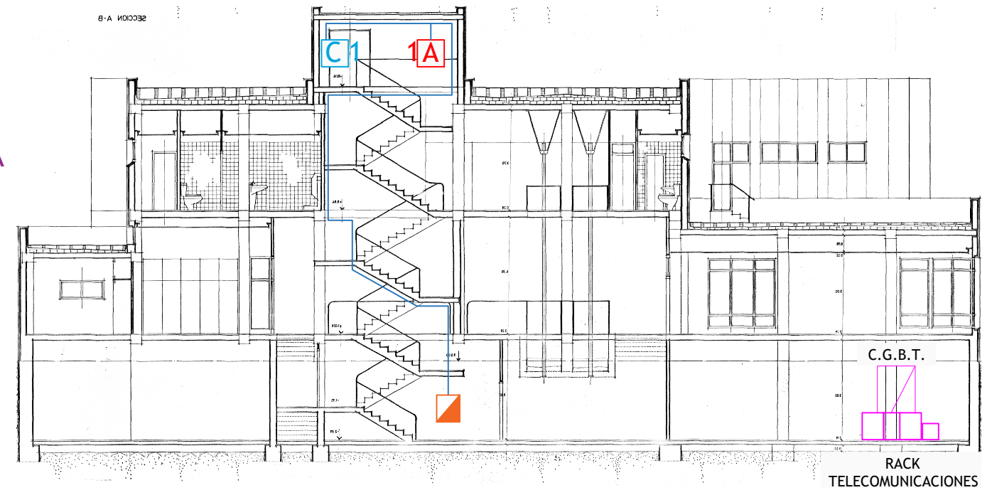
SECCIÓN A-A Escala = 1/200
