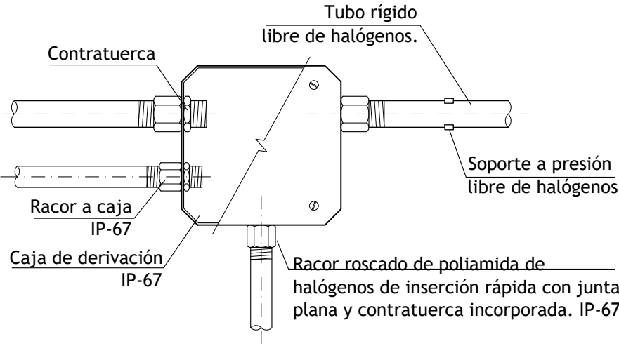
CAJA DERIVACIÓN Escala= 1/5
