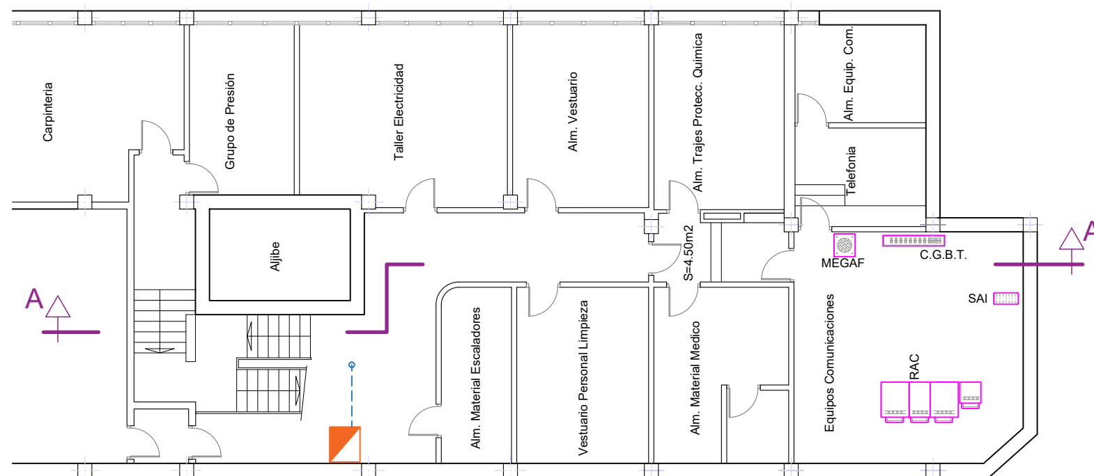
PLANTA SÓTANO Escala = 1/150
