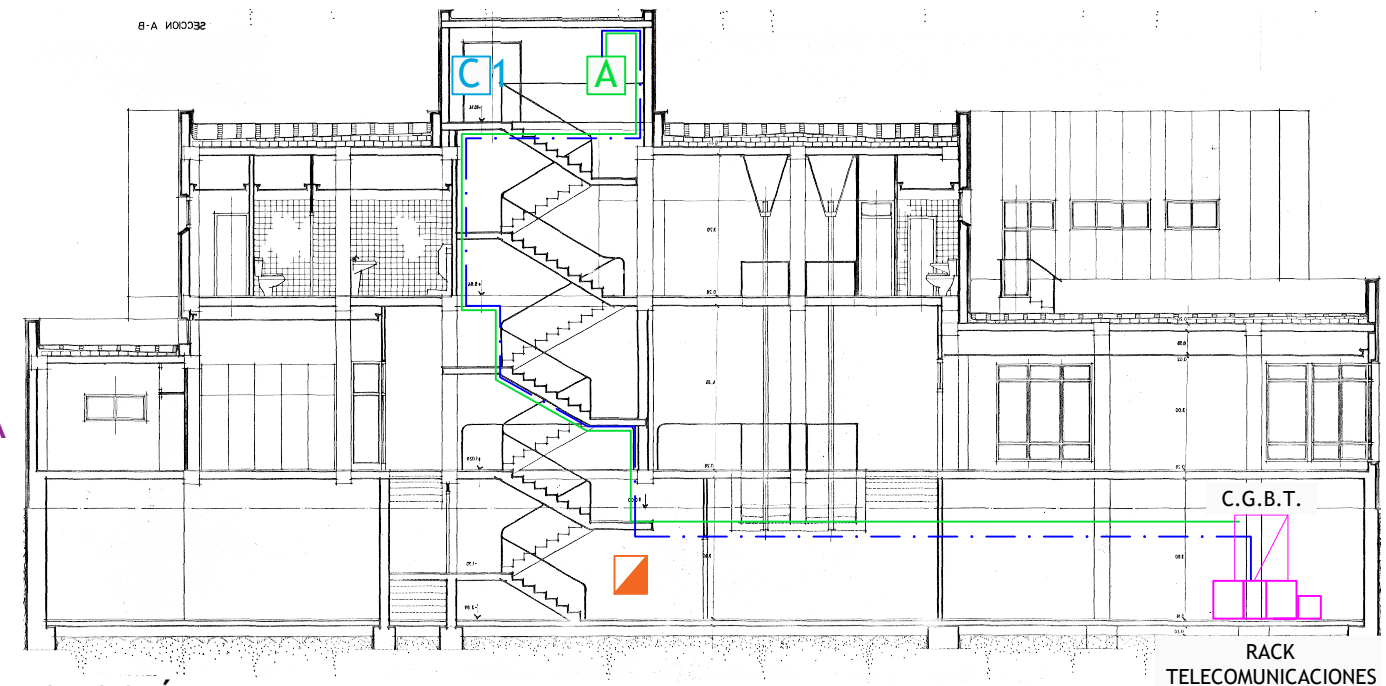
SECCIÓN A-A Escala = 1/200
