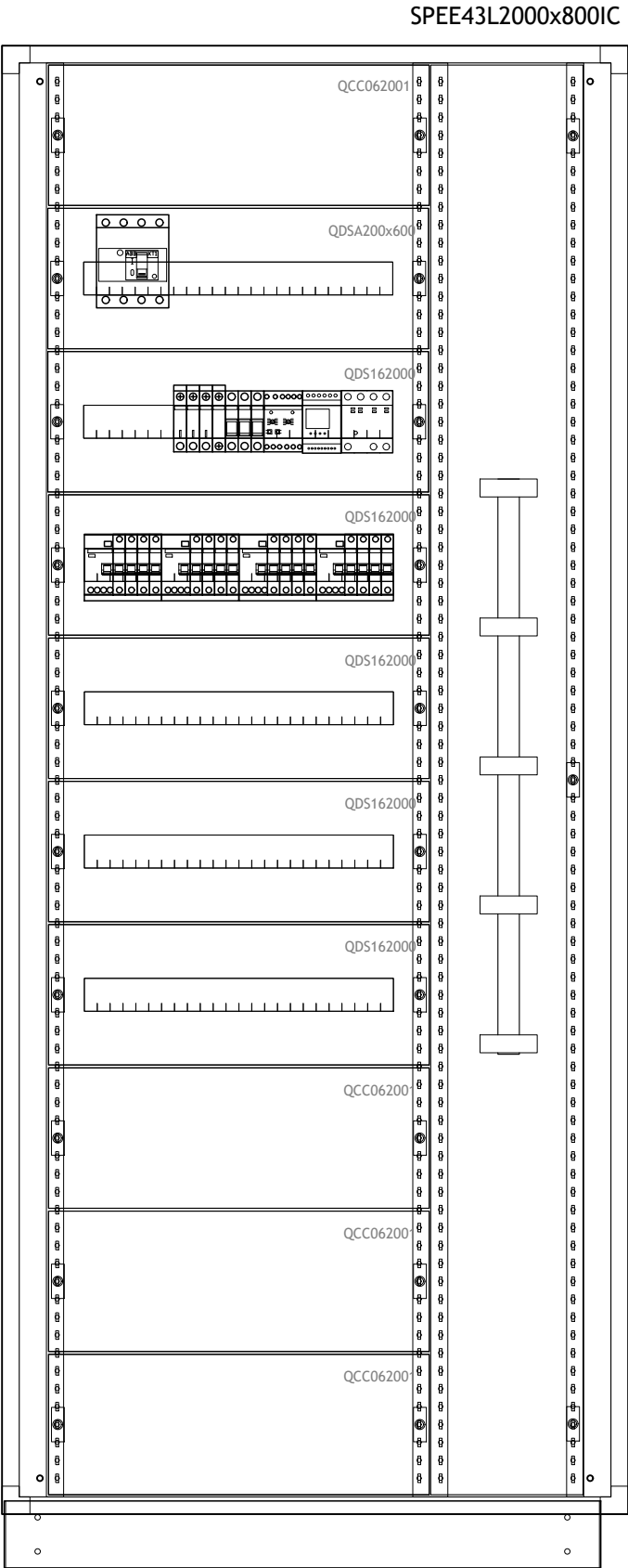
CUADRO DE ALTERNA Escala= 1/10
