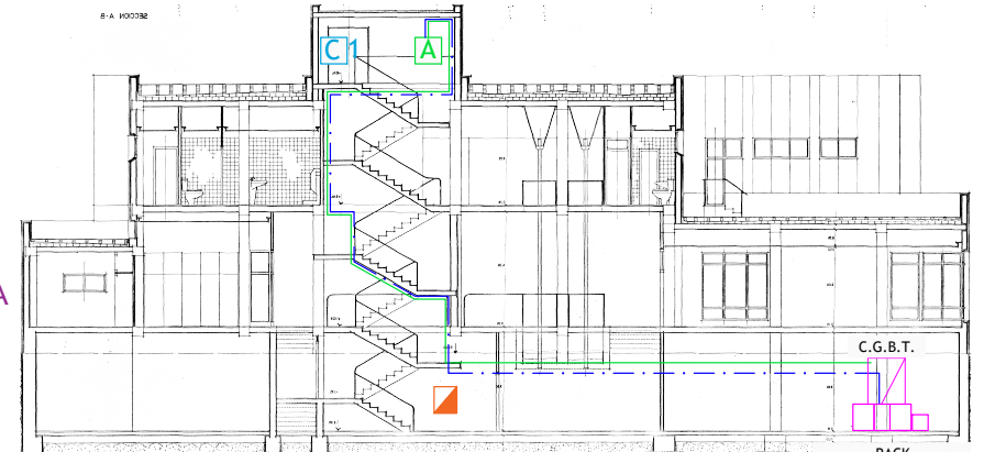
SECCIÓN A-A Escala = 1/200
