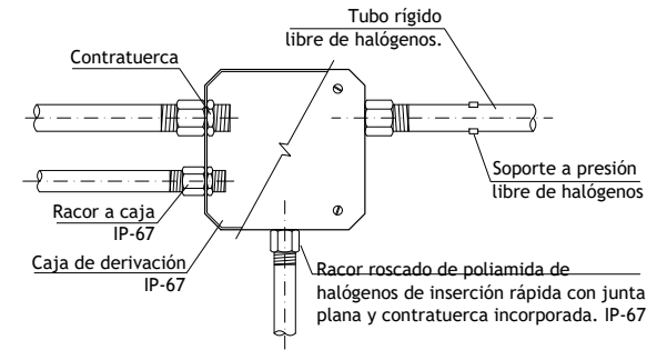
CAJA DERIVACIÓN
