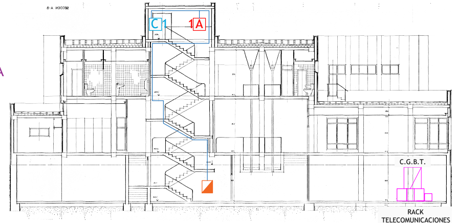
SECCIÓN A-A Escala = 1/200
