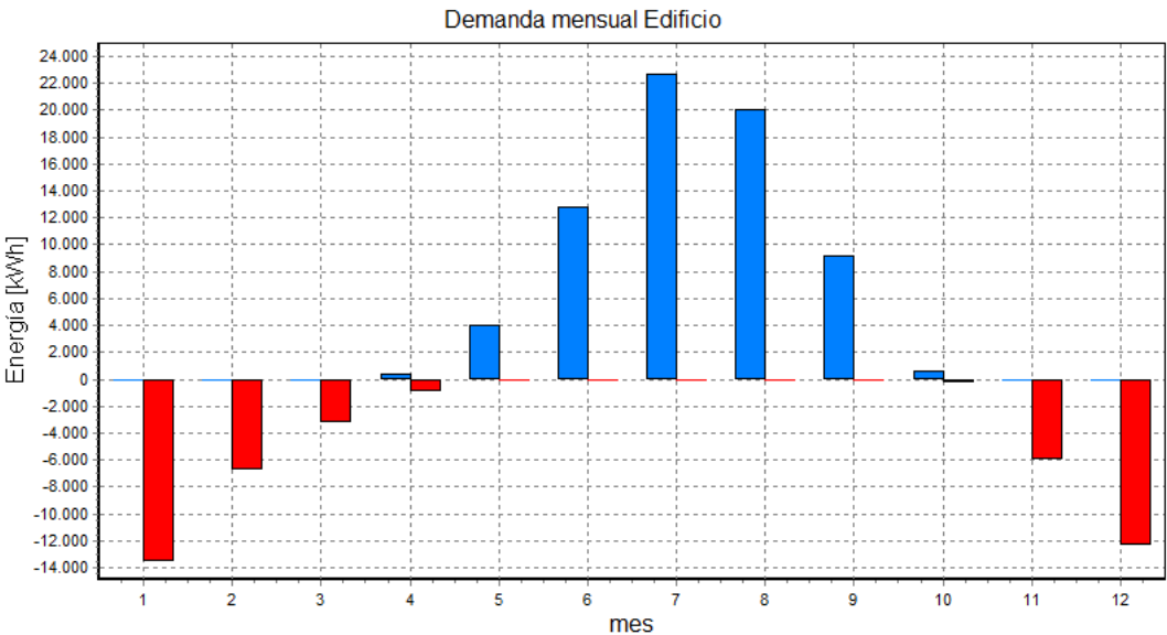
Gráfico de demanda del edificio
