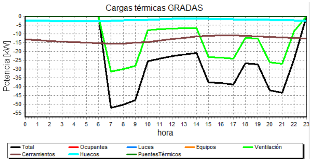
Gráfico de cargas del elemento
