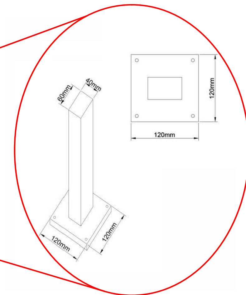
REPLANTEO DE POSTES. TAMAÑO CIMENTACIÓN Y PLACAS DE ANCLAJE DE POSTES
