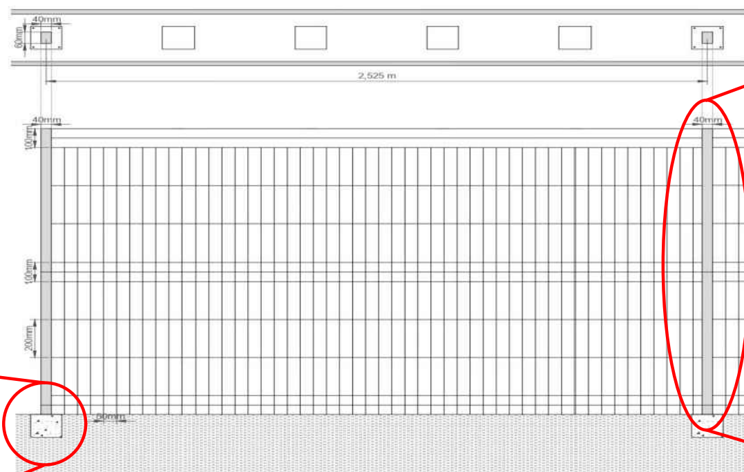
REPLANTEO DE POSTES. TAMAÑO CIMENTACIÓN Y PLACAS DE ANCLAJE DE POSTES
