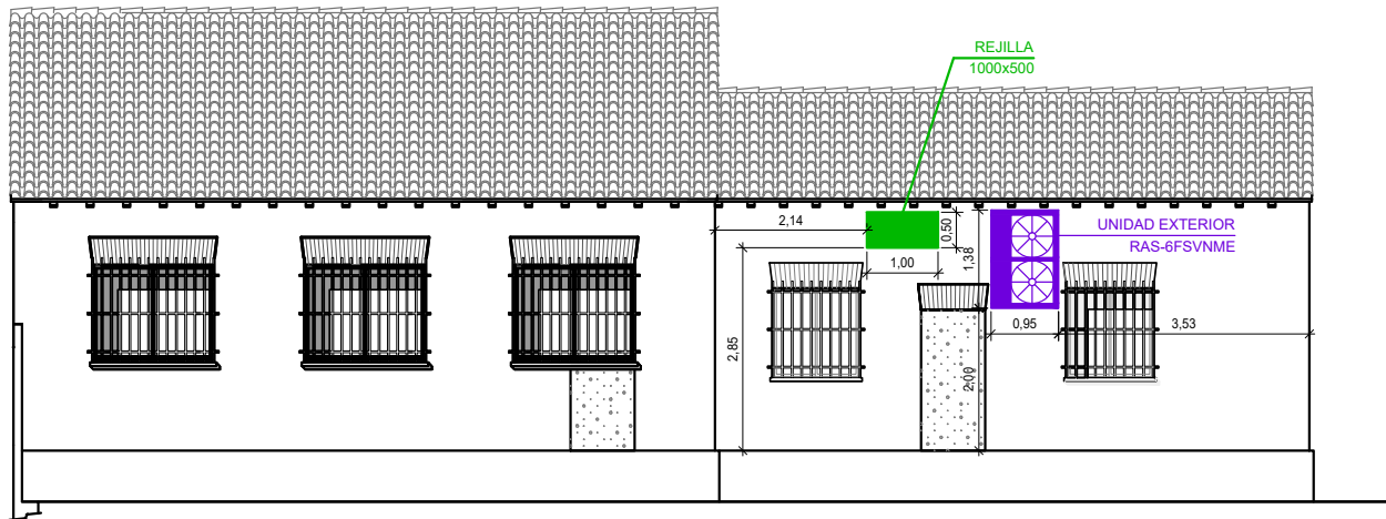
ALZADO POSTERIOR (SUR)
