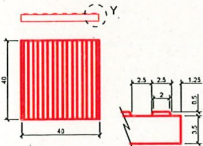
BALDOSA 40x40x3,5 cm
