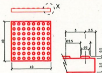
BALDOSA 40x40x3,5 cm (8x8) tacos COTAS EN cm
