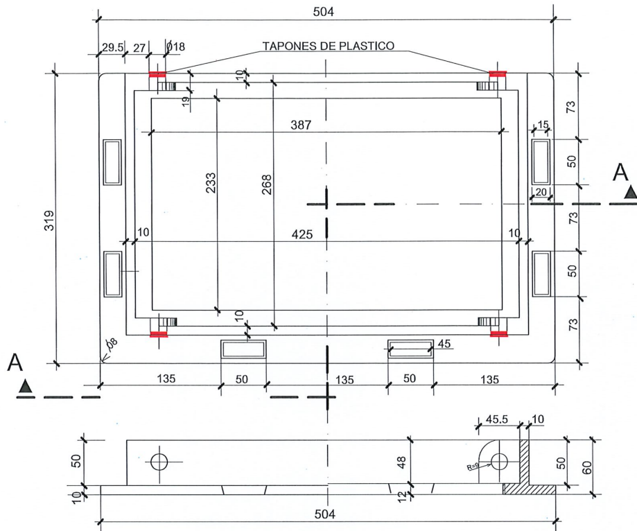
ALZADO-SECCION A-A
