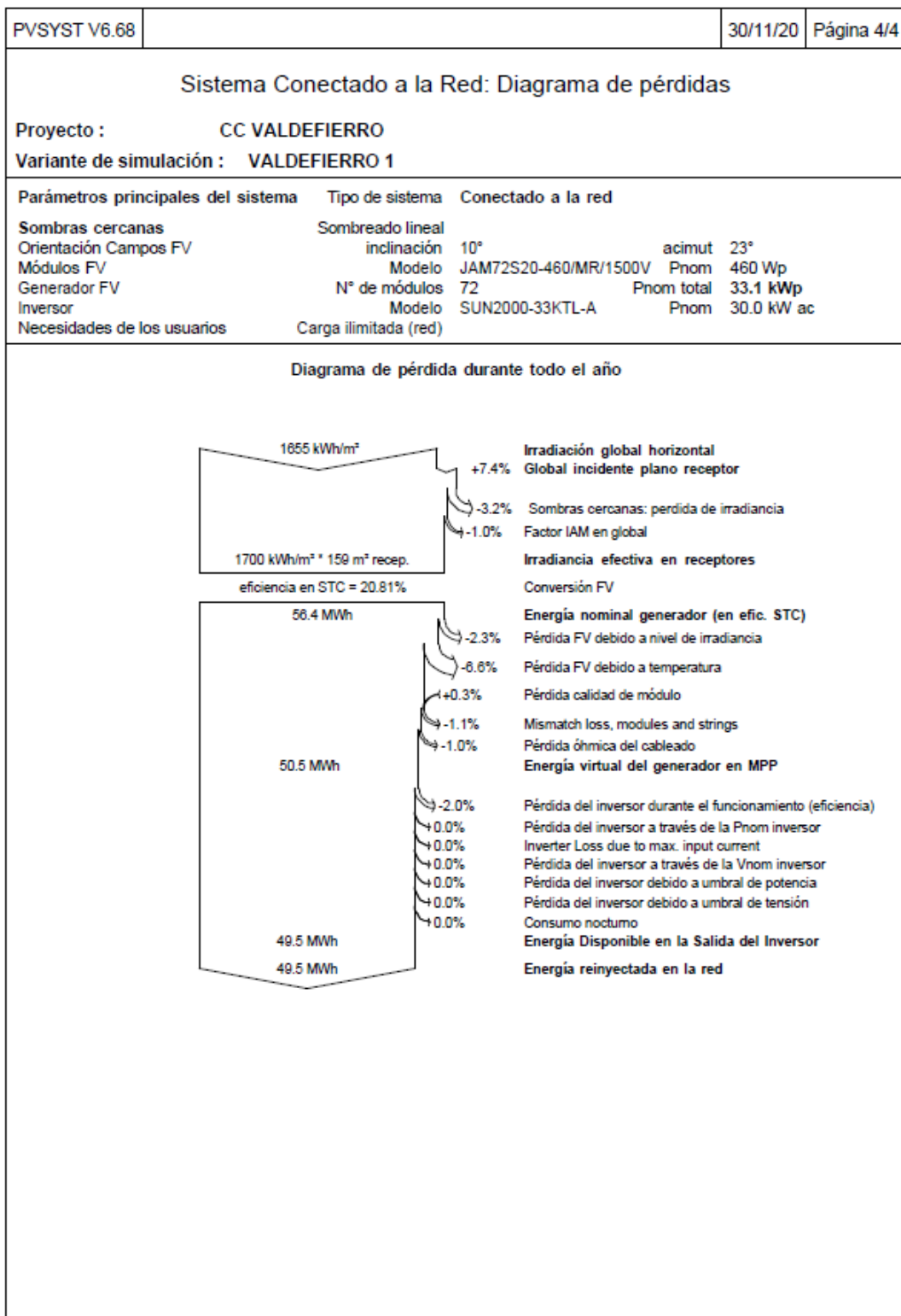
Diagrama 1: distribución de pérdidas de la instalación simulado con PVSYST
