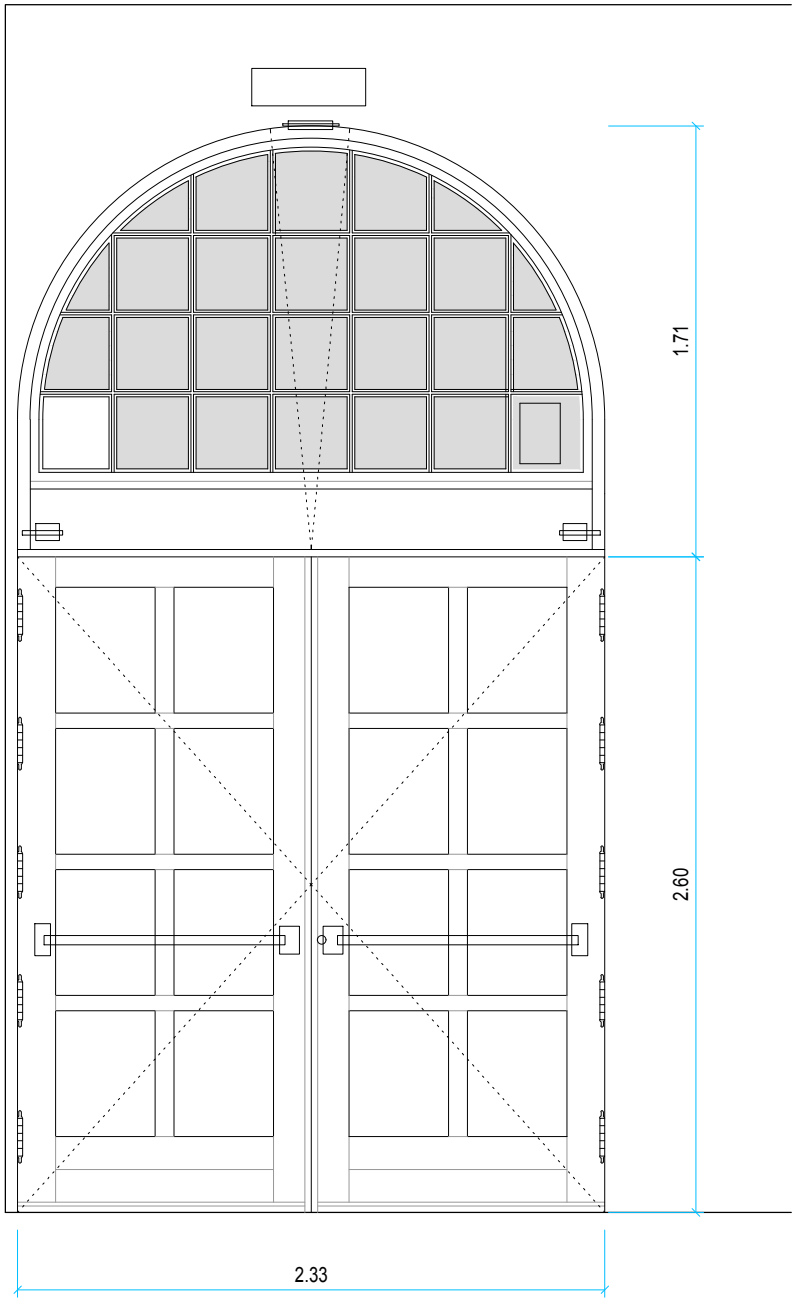
ALZADO INTERIOR E. 1/30
