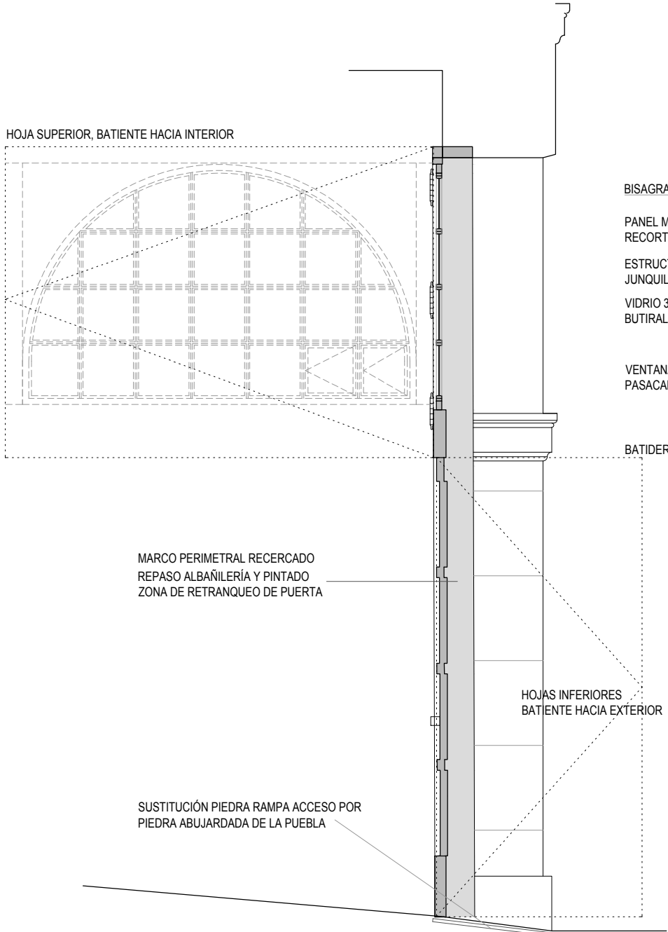
SECCIÓN E. 1/30
