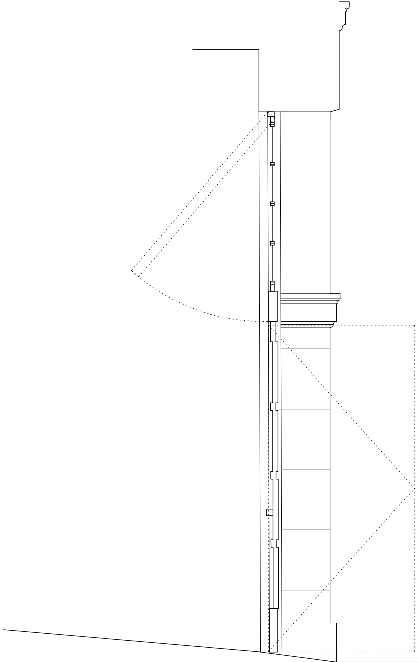
SECCIÓN E. 1/30
