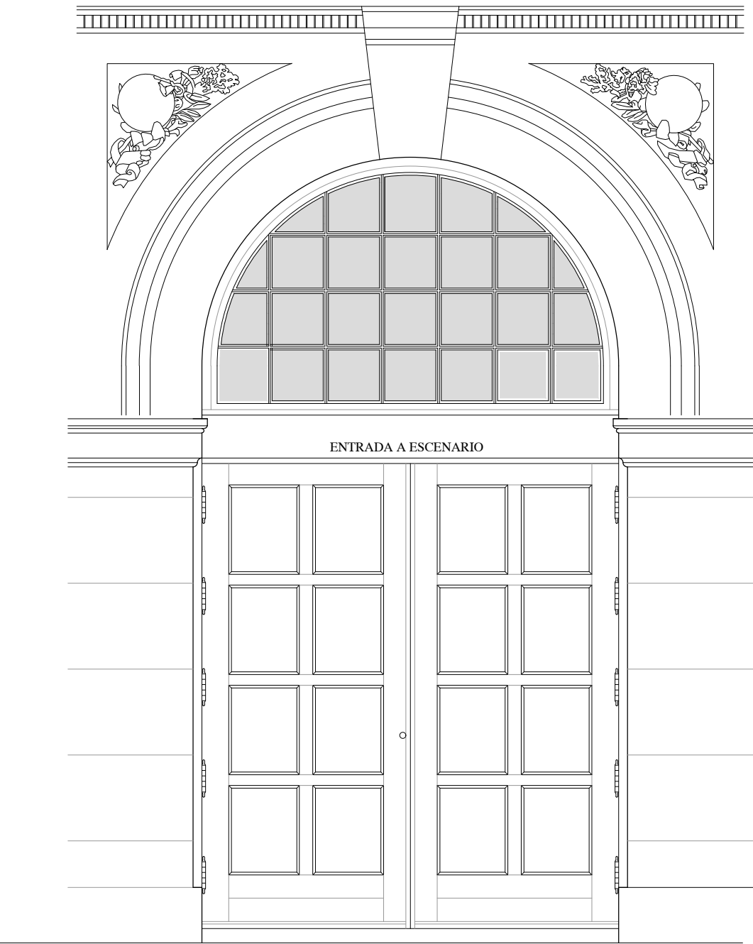
ALZADO EXTERIOR E. 1/30
