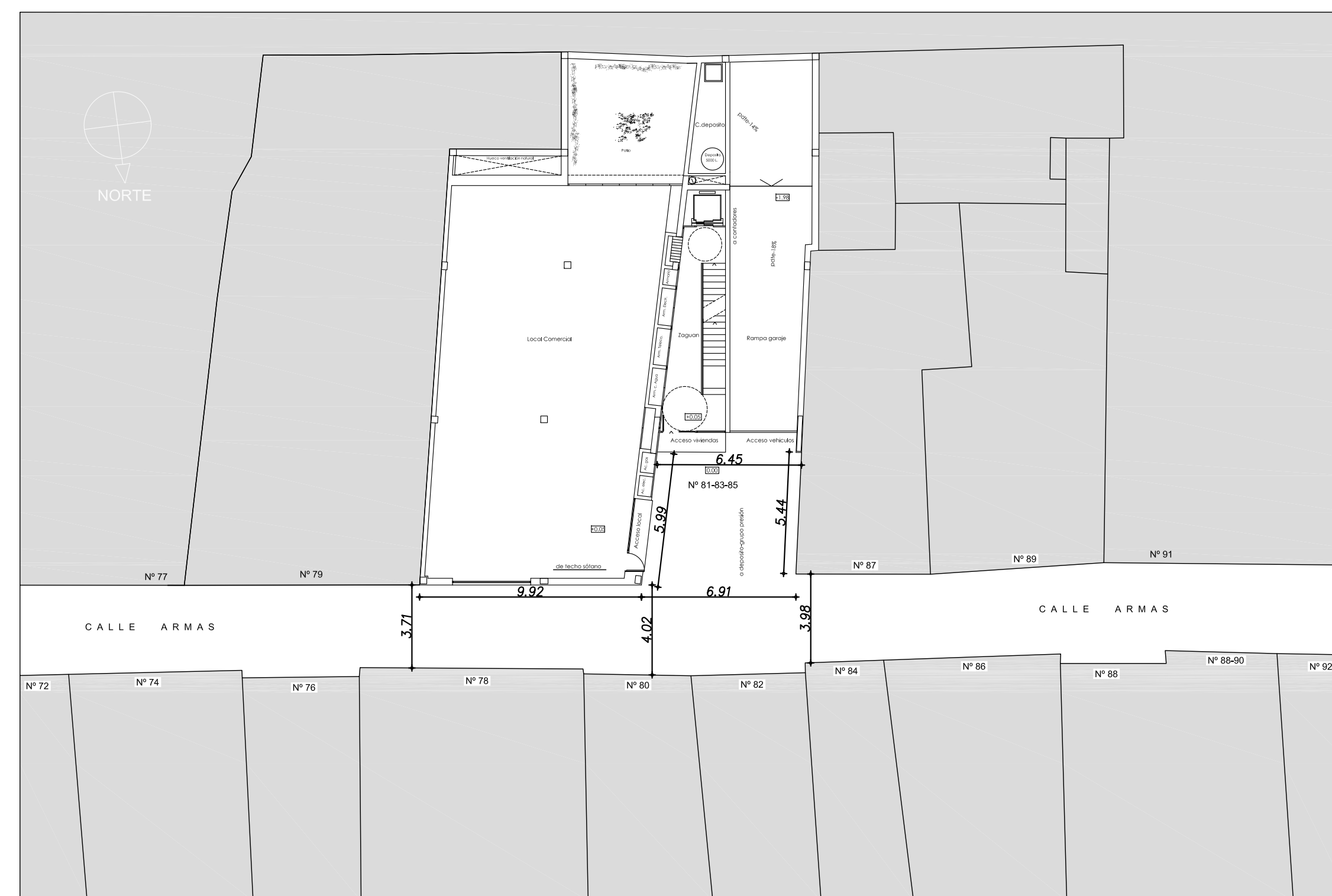
PLANO DE SITUACION ESCALA 1/200
