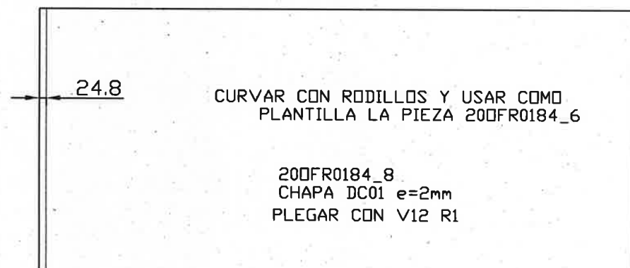
200FR0184_7 CHAPA DC01 e=2mm PLEGAR CON V12 R1
