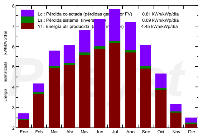
Producciones normalizadas (por kWp instalado): Potencia nominal 25.30 kWp
