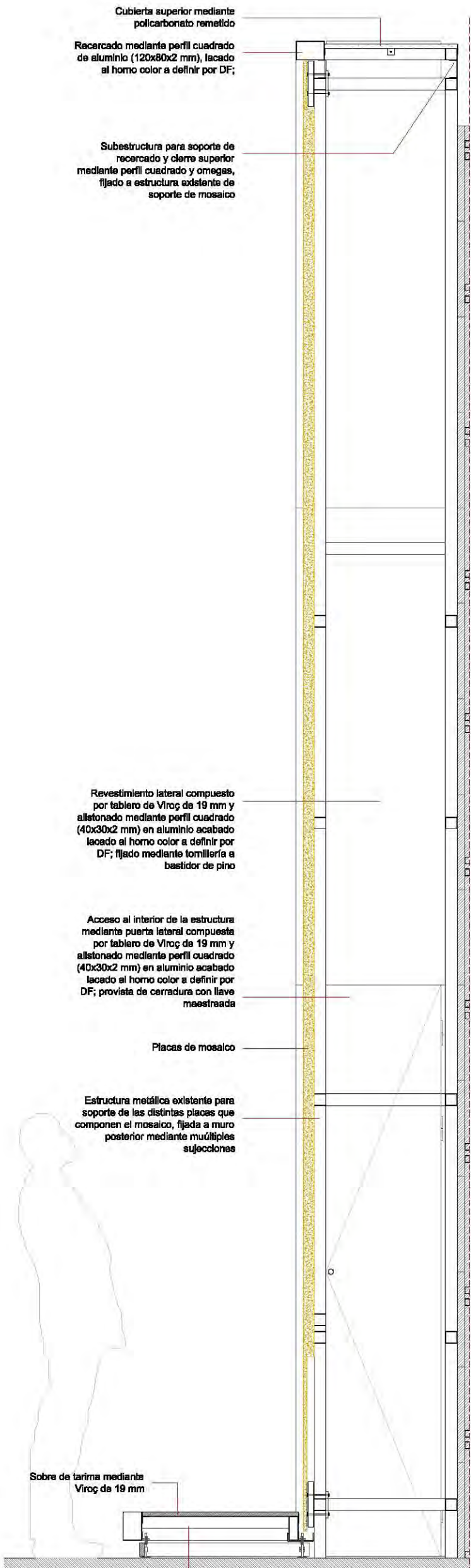
Sección S2 e. 1/20
