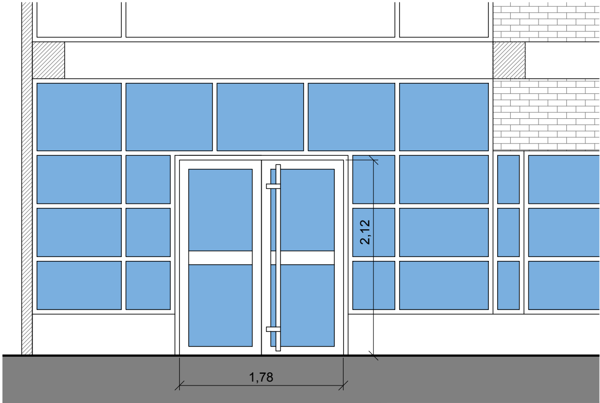
VISTA D - D' (SUSTITUIR HOJAS MÓVILES) E=1:40
