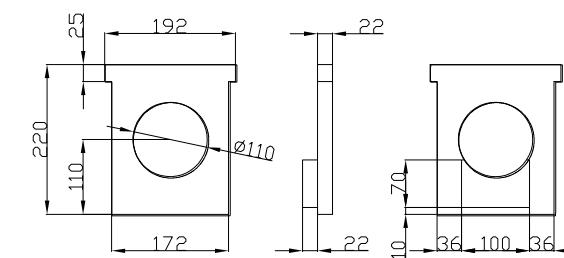
DETALLE PIEZA PARA ENCOFRAR
