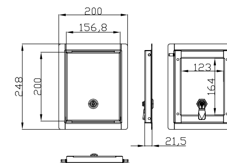
DETALLE PUERTA DE ZOCALO
