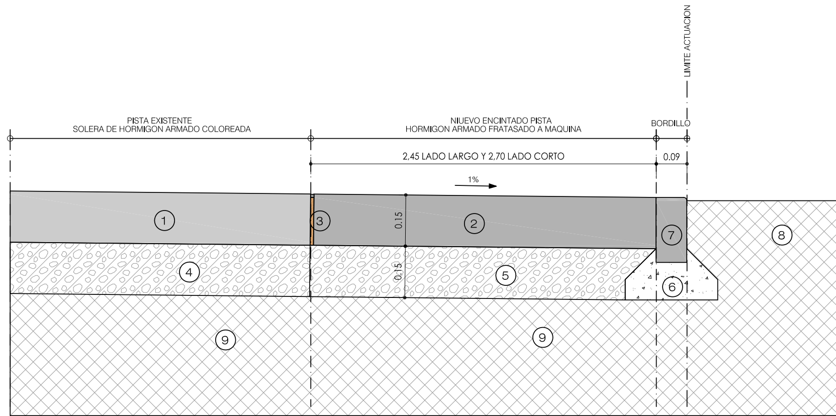
SECCIÓN TIPO ESCALA 1/10
