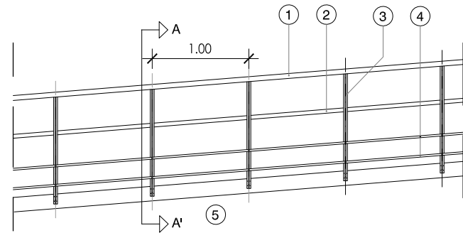
ALZADO E. 1/50
