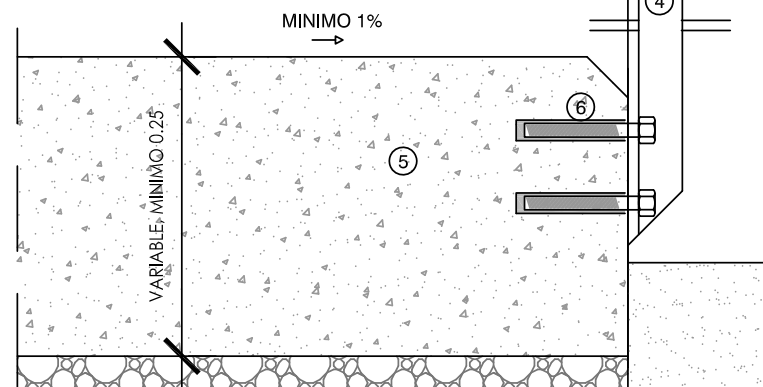
DETALLE E. 1/5
