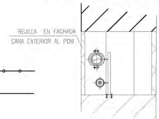
DETALLE N° 3: UBICACIÓN DEL ACTUAL TUBERIA DE GAS Y CABLE DE PULSOS DENTRO DE CAMARA EN EL PDM
