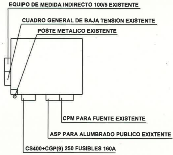
INSTALACION DE ENLACE ACTUAL
