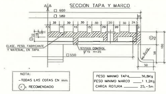
MARCO Y TAPA CUADRADO DE 60 cm.
