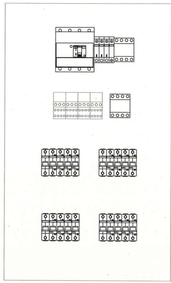
Armario mural SR2 1000x600x250 (instalar un carril DIN extra para futuras ampliaciones)
