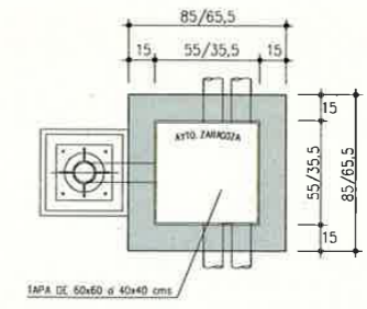
PAREDES DE ARQUETAS DE HORMIGON HM-30/P/22/I o I+Qb SEGUN TIPO DE TERRENO ARQUETAS DE DERIVACION
