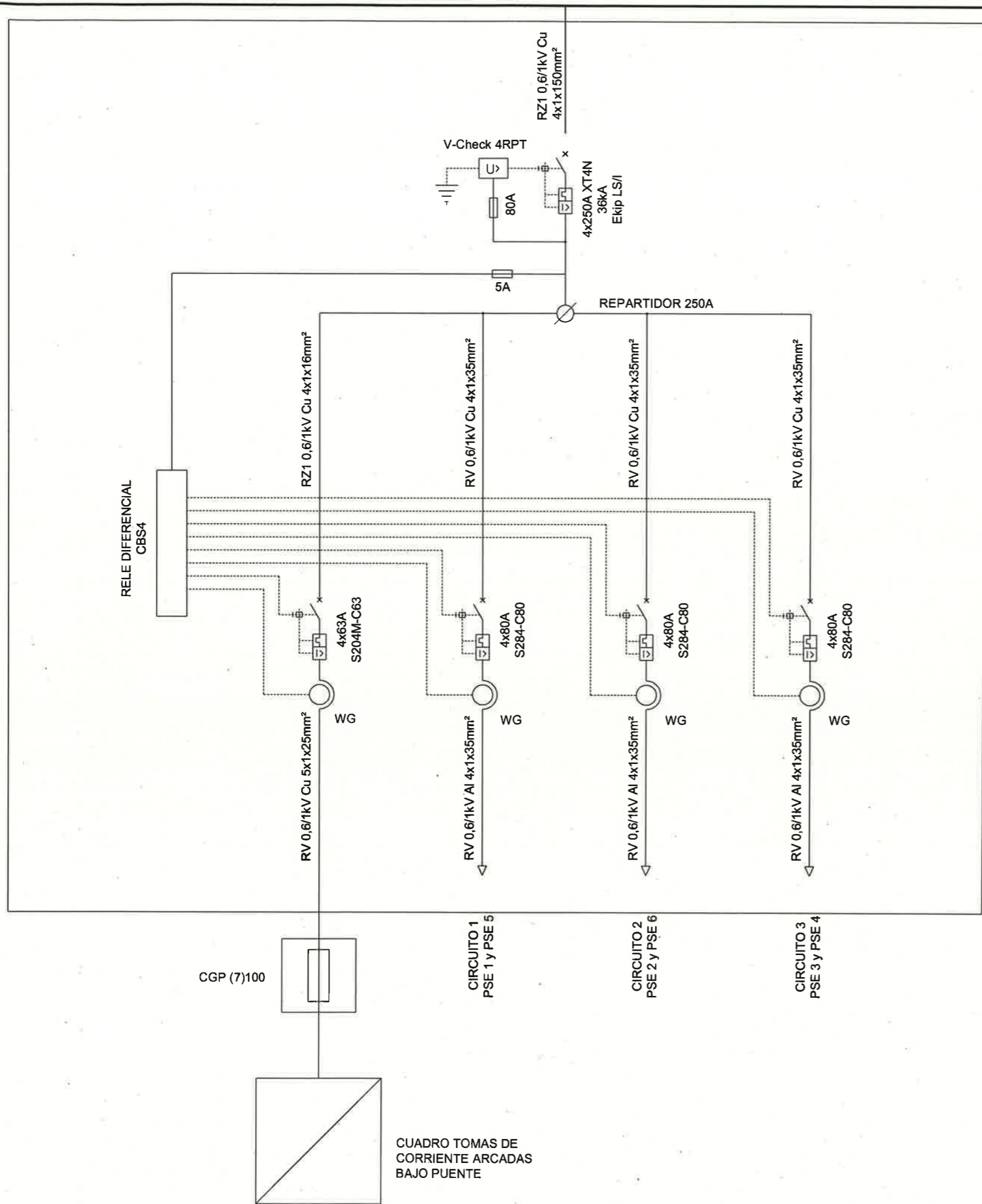
ESQUEMA UNIFILAR. CUADRO PRINCIPAL
