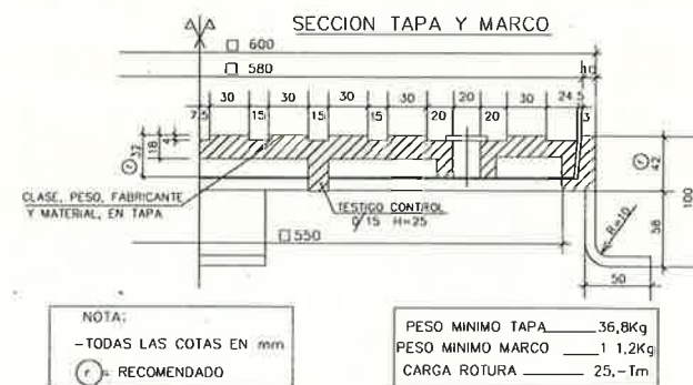
MARCO Y TAPA CUADRADO DE 60 cm.
