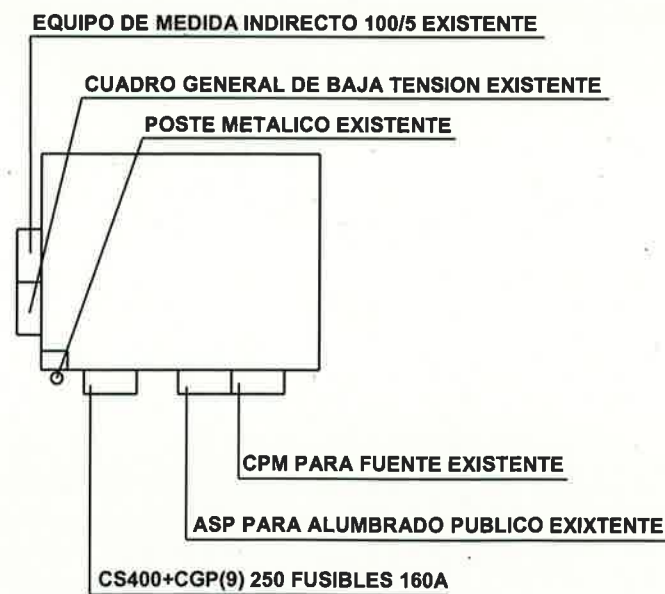
INSTALACION DE ENLACE ACTUAL
