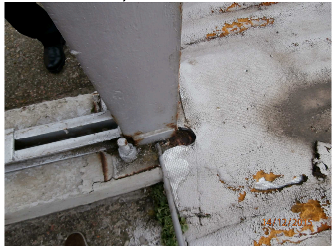
Daños en estructura cubierta oeste
