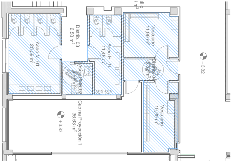
PLANTA PRIMERA_ASEOS TORRE Y VESTUARIOS
