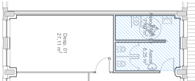
PLANTA SEGUNDA_ASEOS ADMINISTRACION
