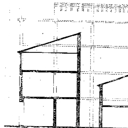
Sección longitudinal
