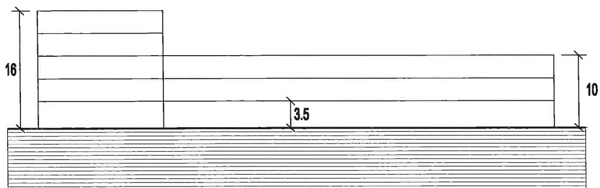
SECCIÓN ORIENTATIVA A con planta baja diáfana
