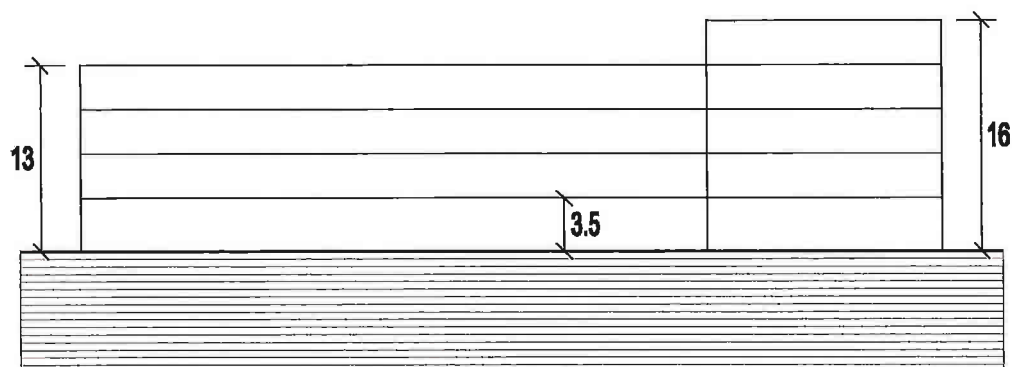
SECCIÓN ORIENTATIVA B con planta baja diáfana
