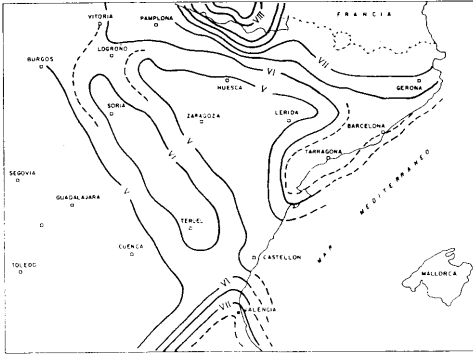
Figura I.6.3.: Riesgo sísmico de probabilidad 0,001.
