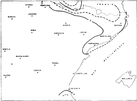
Figura I.6.1.: Riesgo sísmico de probabilidad 0,01.
