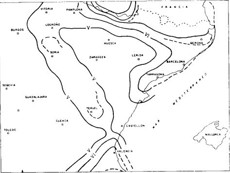
Figura I.6.2.: Riesgo sísmico de probabilidad 0,002.
