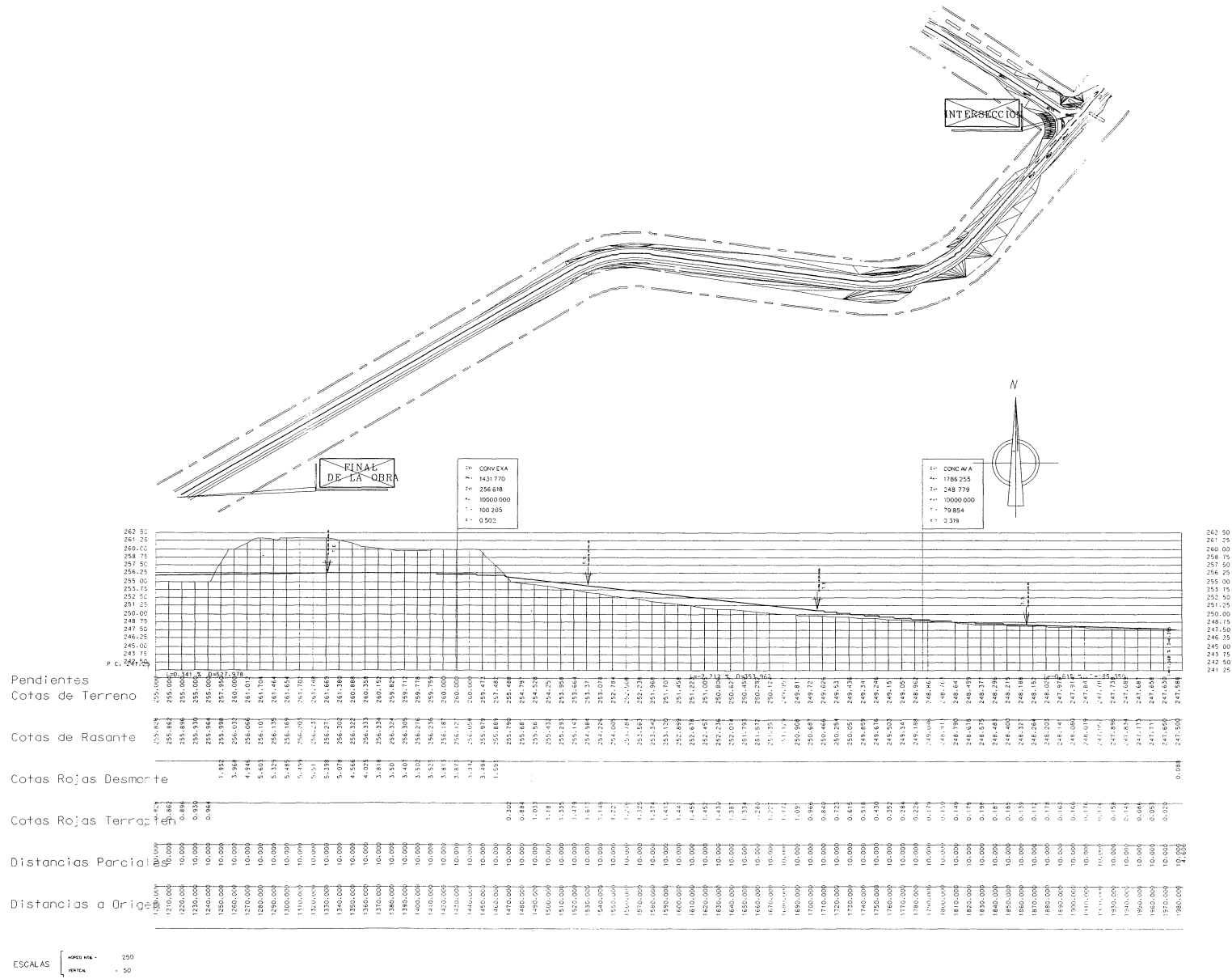
PERFIL LONGITUDINAL ALTERNATIVA A LAS TRES SOLUCIONES (SOBRE PERFIL SOLUCION 1 - 2)
