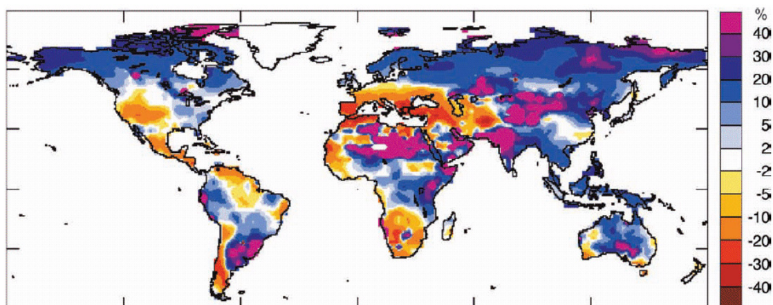
Figura 1. Mapa mundial de variación porcentual de la escorrentía el escenario A1 de SRES, elaborado a partir de los resultados de 12 modelos de clima (IPCC, 2007)
