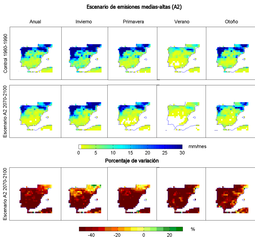
Figura 2. Resultado de las simulaciones de escorrentía en el proyecto PRUDENCE para el escenario de emisiones A2 (media de varios modelos)
