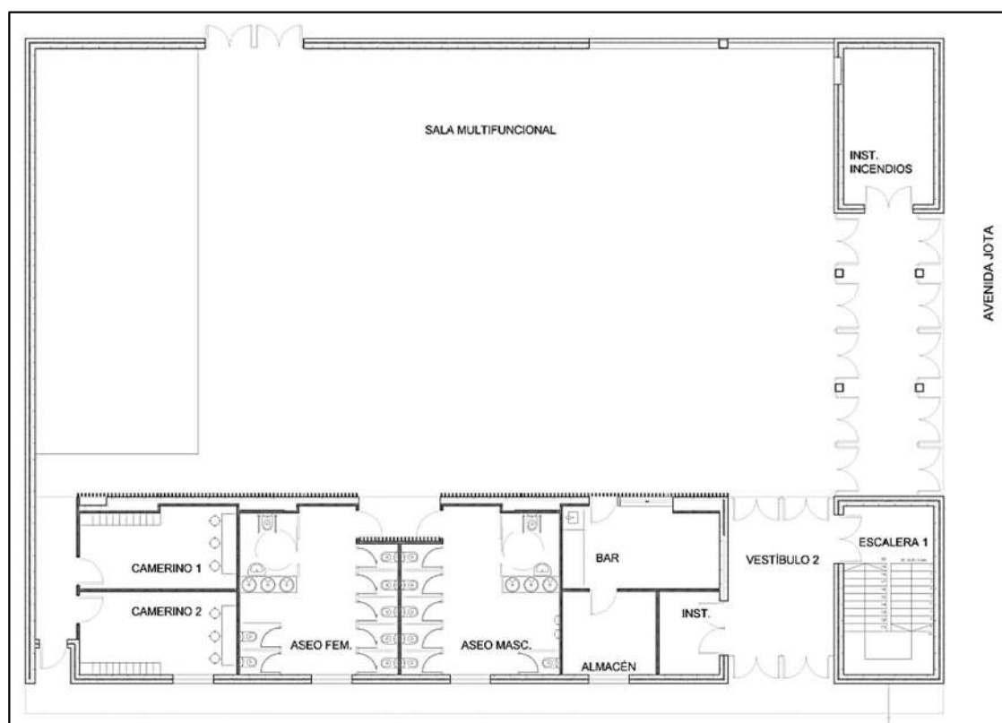
Plano de Planta Baja
