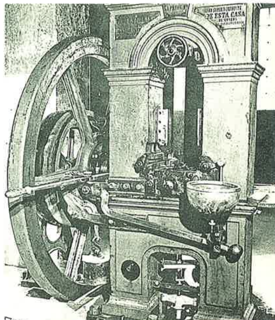
Prensa de tipo Le Thonelier, usada en la Fábrica Nacional de Moneda y Timbre
