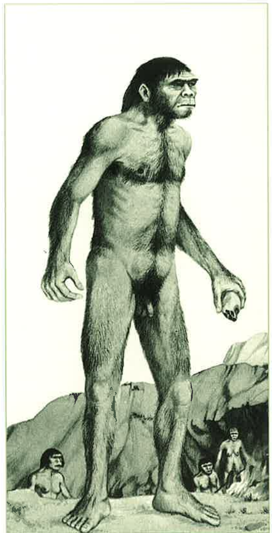
Homo erectus
