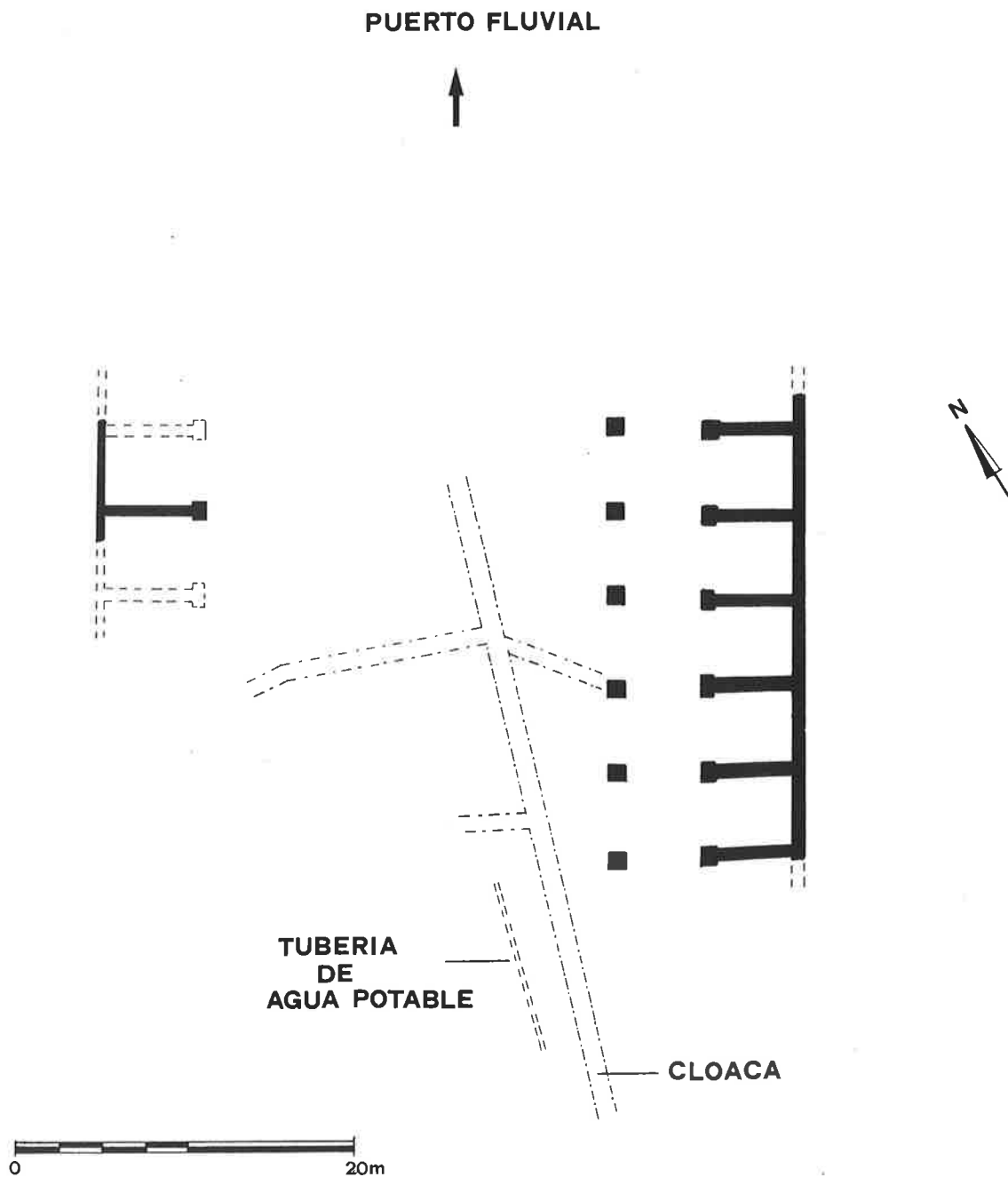
Figura 45 Plano nº 2.
