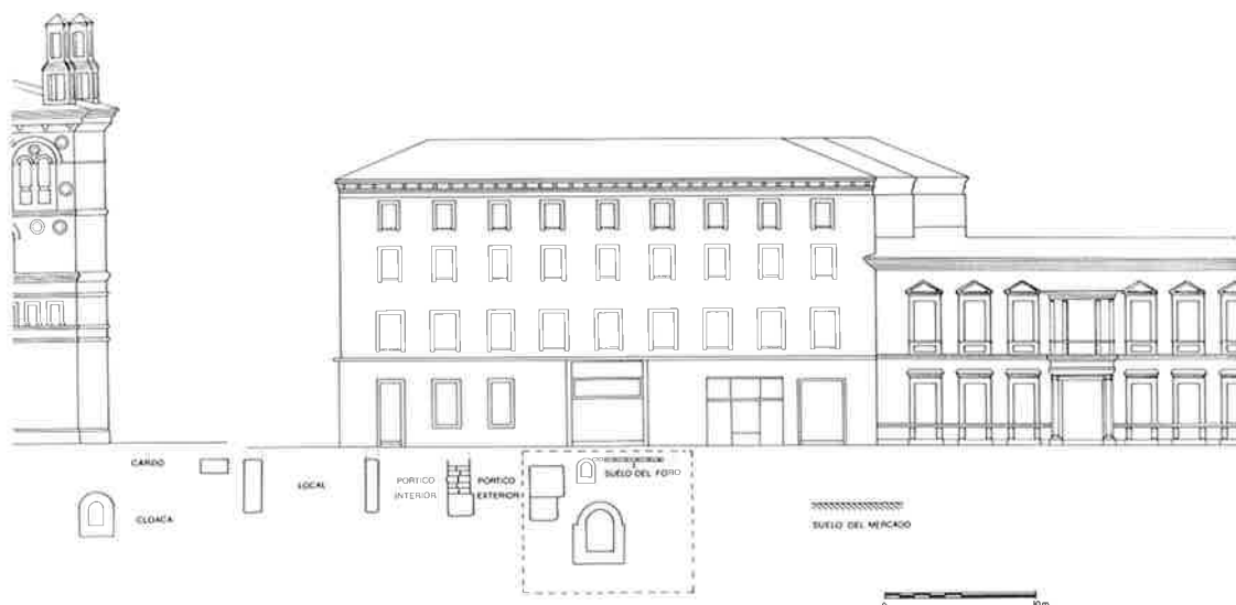
Figura 63 Corte de la plaza de La Seo.
