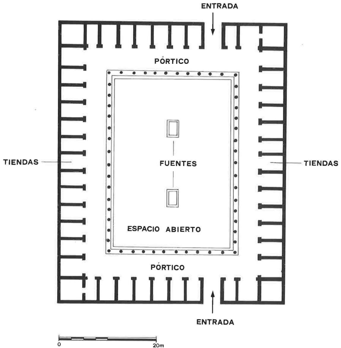
Figura 45 Plano nº 1.
