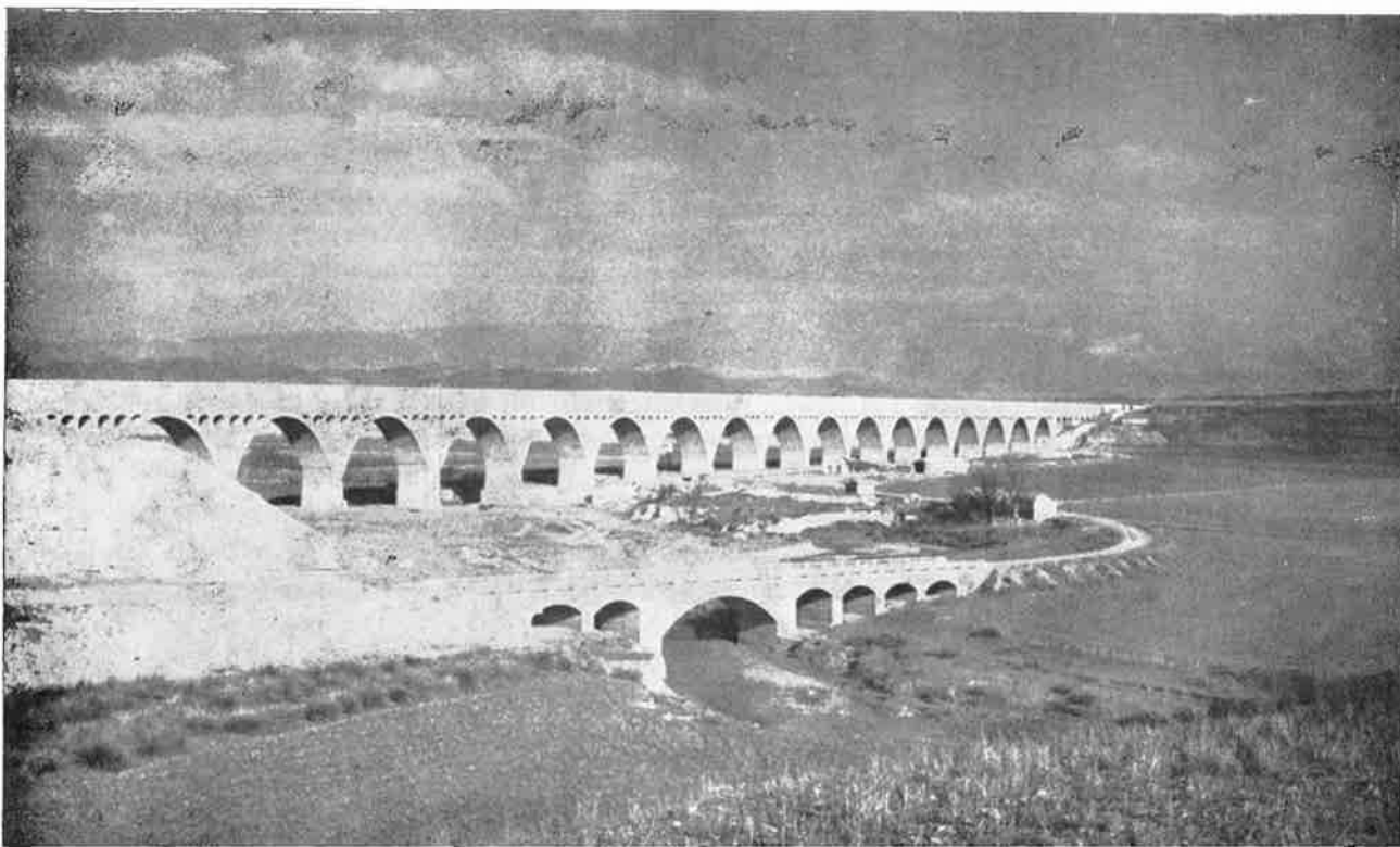
Canal de las Bardenas. Acueducto de Onsella.
