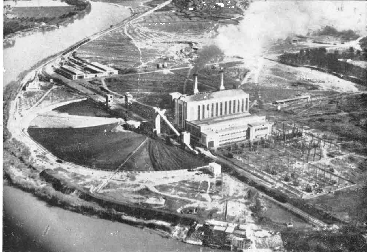
Central térmica Escatrón.
