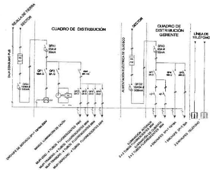
ESQUEMA ELÉCTRICO
