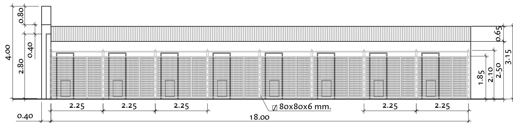
ALZADO LATERAL
