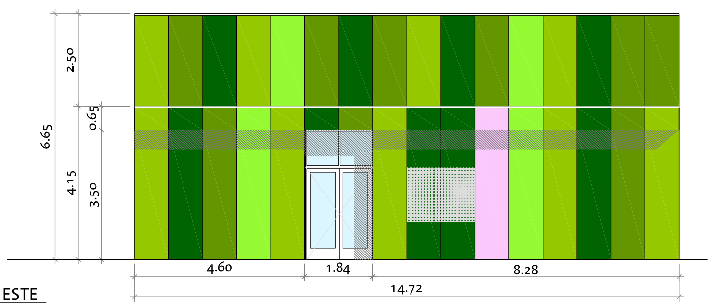
FACAHADA SUR Escala= 1/100
