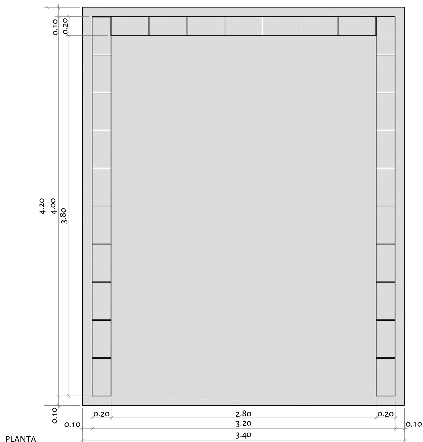
PLANTA
