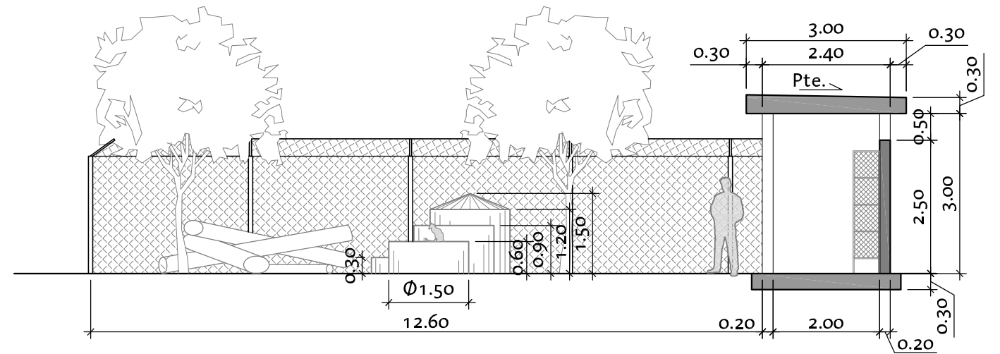
SECCION B-B
