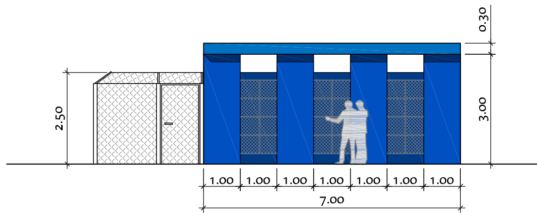
ALZADO-SECCION A-A
