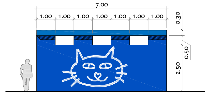
ALZADO "C"
