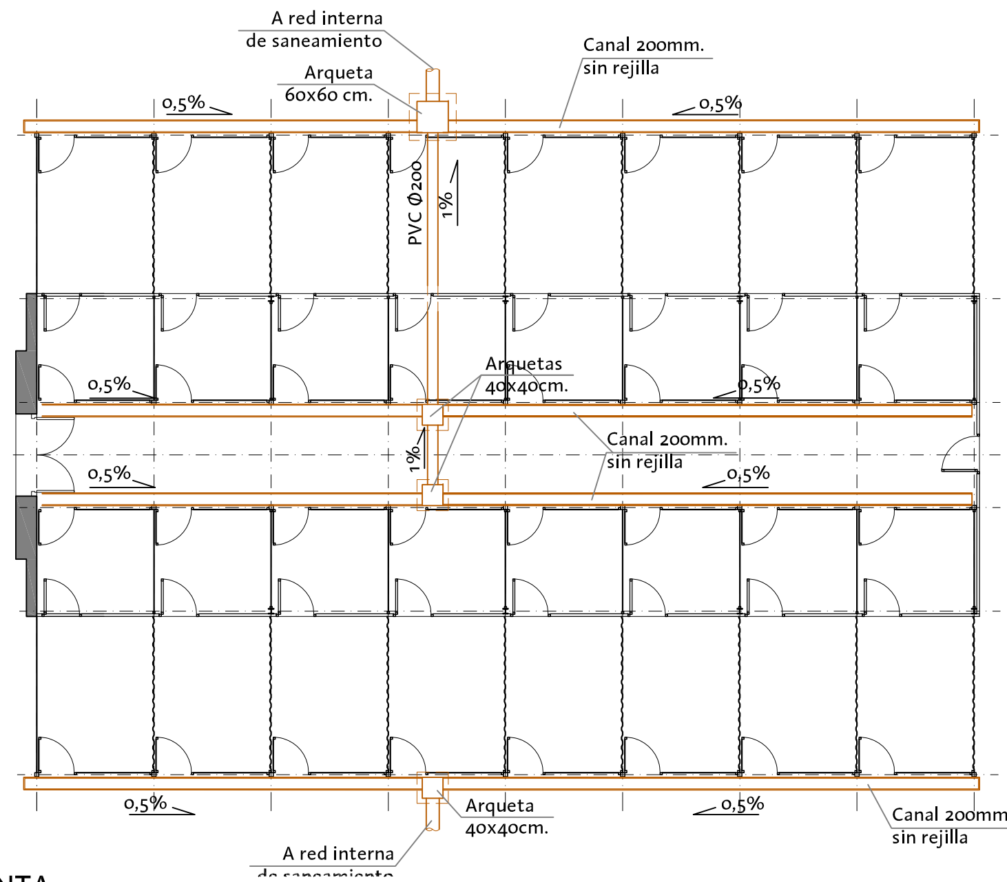
PLANTA
