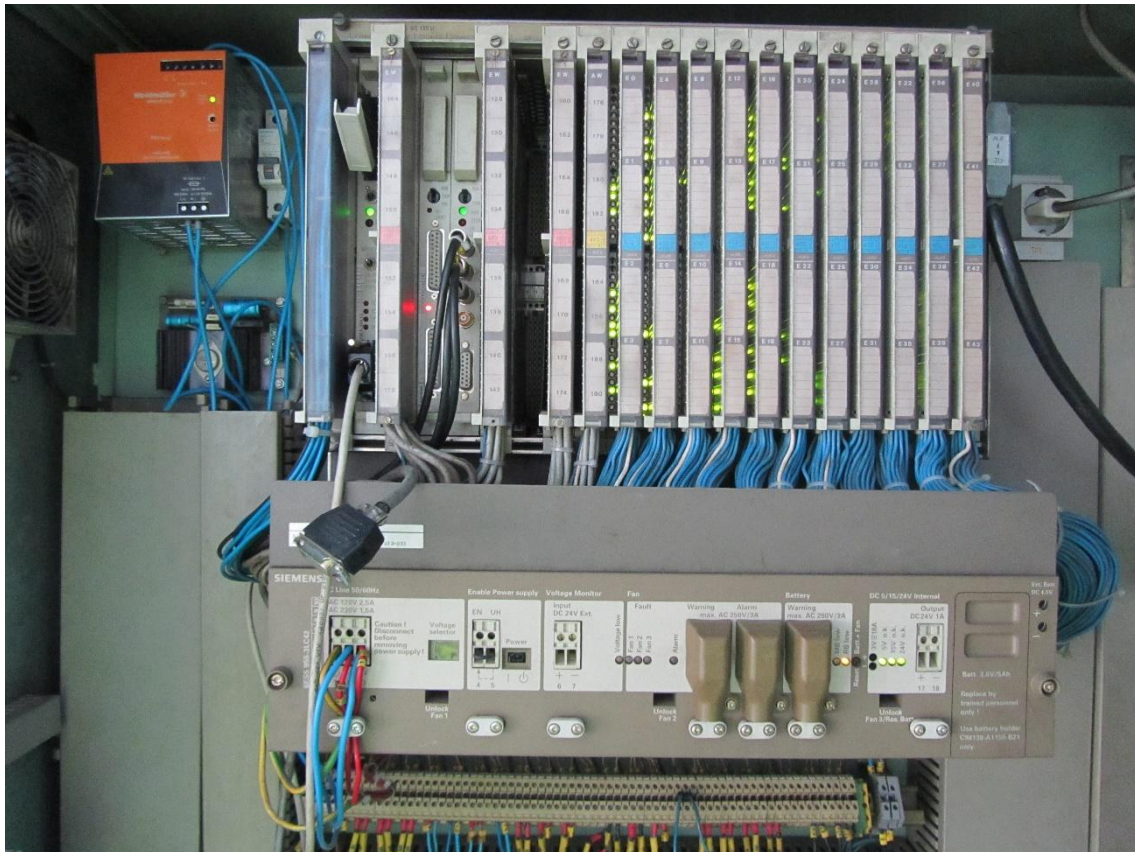
Automata S5 existente.
