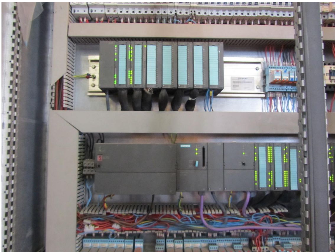
Control Centro de Control de Motores existente.
