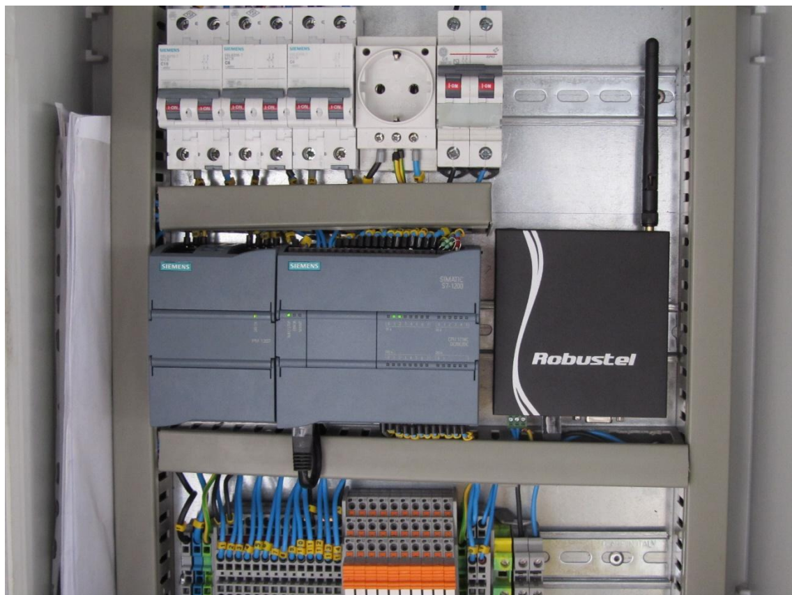
Equipos de telecontrol existente.
