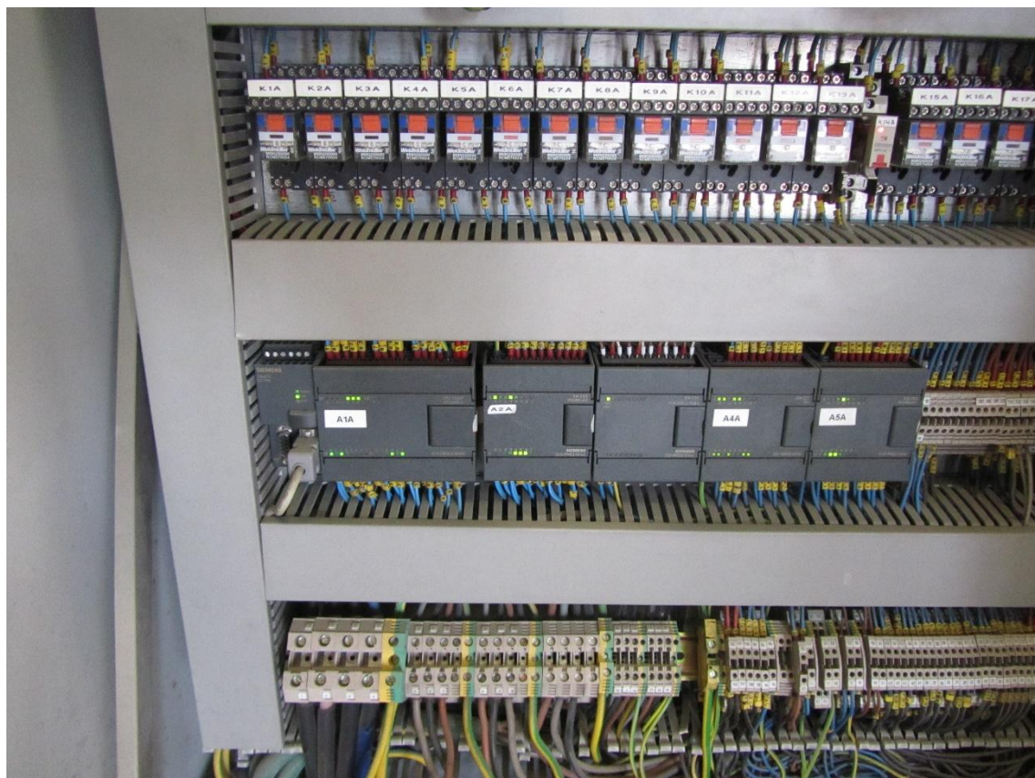
Armario de control de filtros de arena existente.
