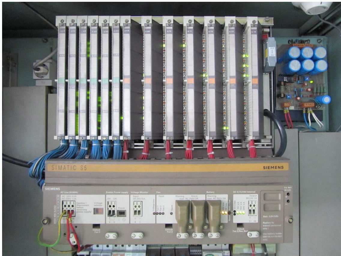
Extensión automática existente.
