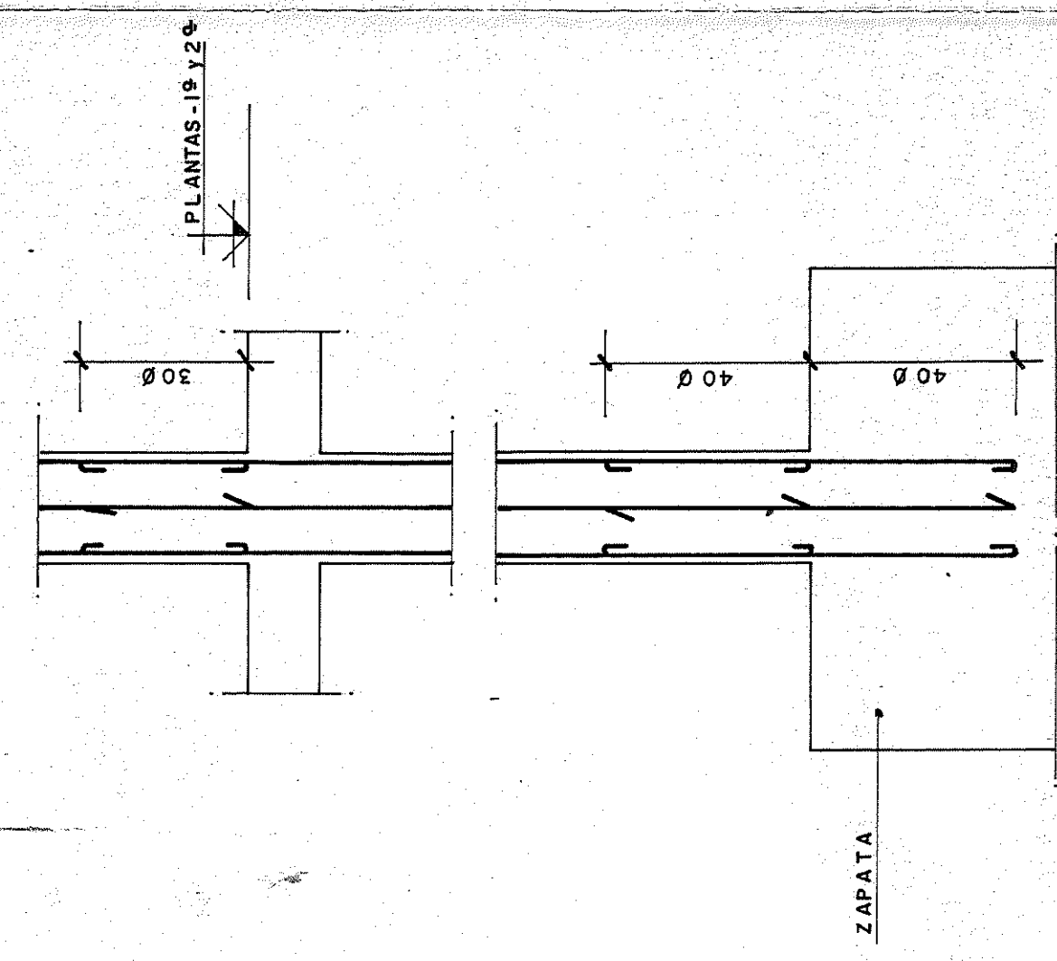
DETALLE DE ANCLAJES DE ARMADURA EN PILARES
