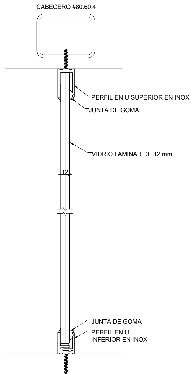
DETALLE DE SECCIÓN DE VIDRIERA FIJA
