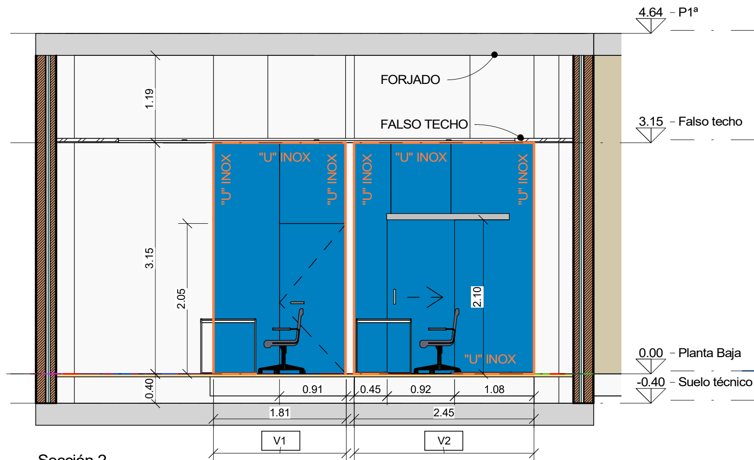
Sección 2 1 : 50
