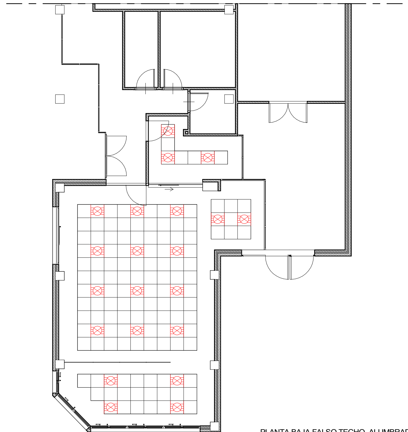
PLANTA BAJA FALSO TECHO. ALUMBRADO 1:100
