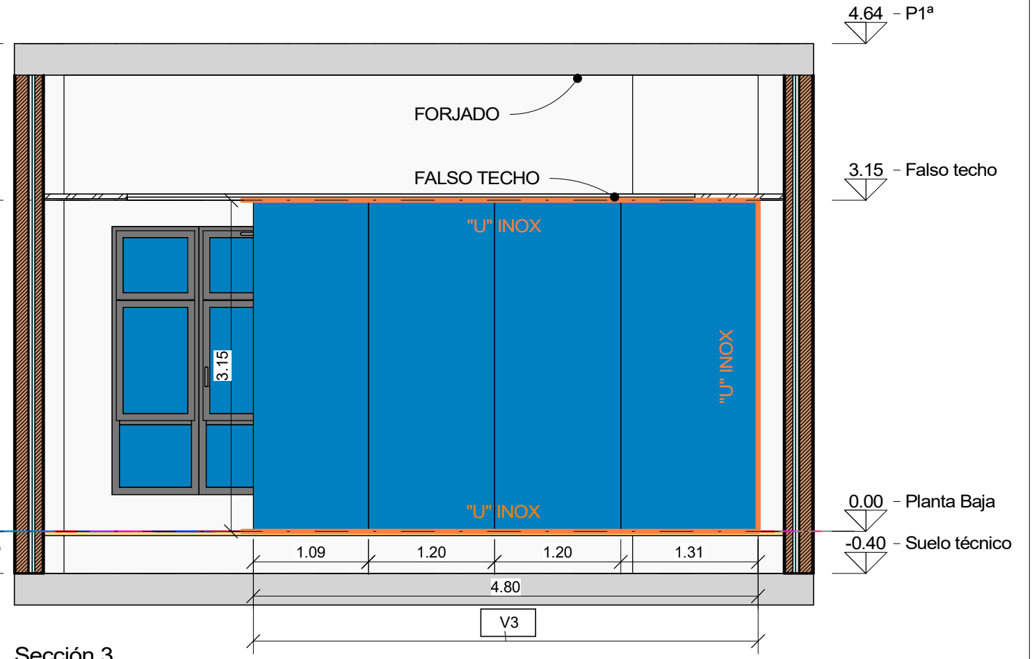
Sección 3 1 : 50
