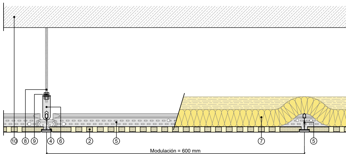
Sección vertical
