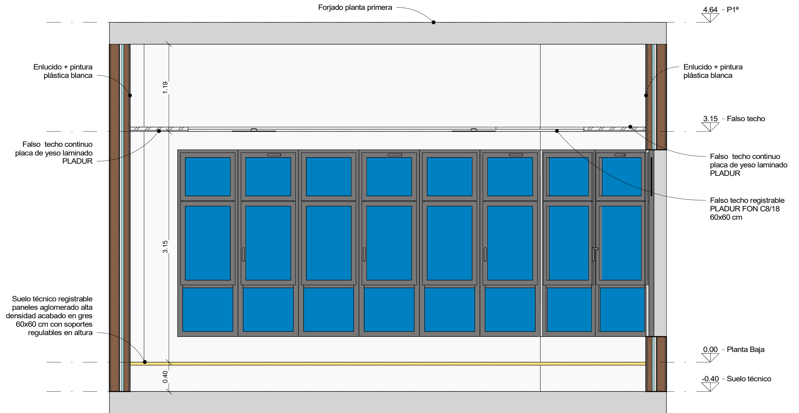
Sección 1 1 : 30
