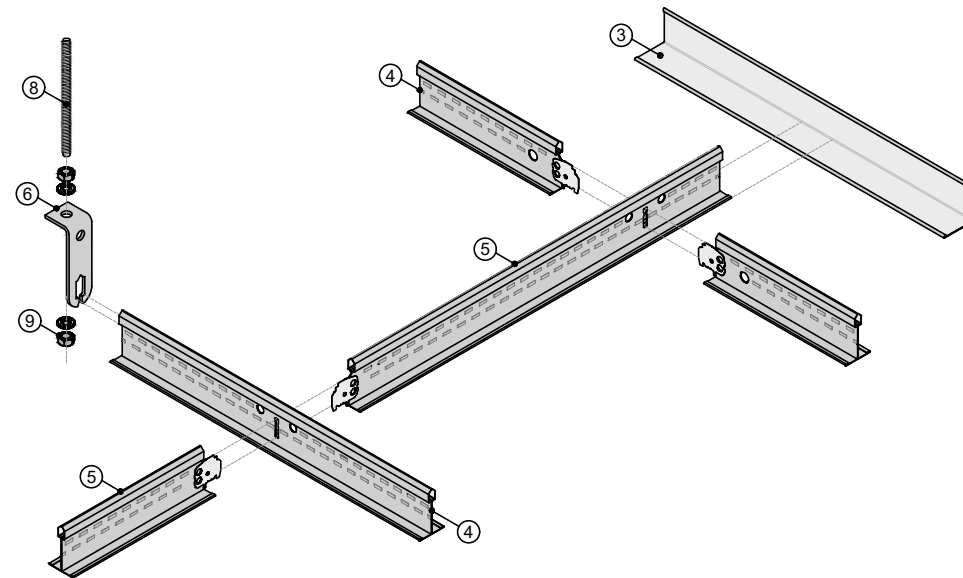
Vista isométrica
