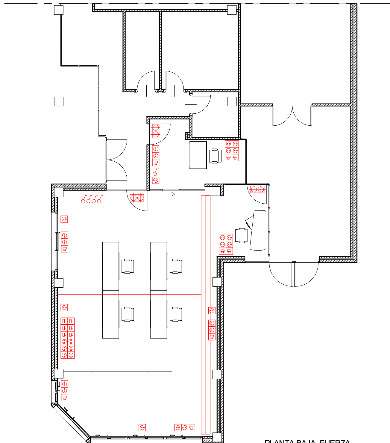
PLANTA BAJA. FUERZA 1:100
