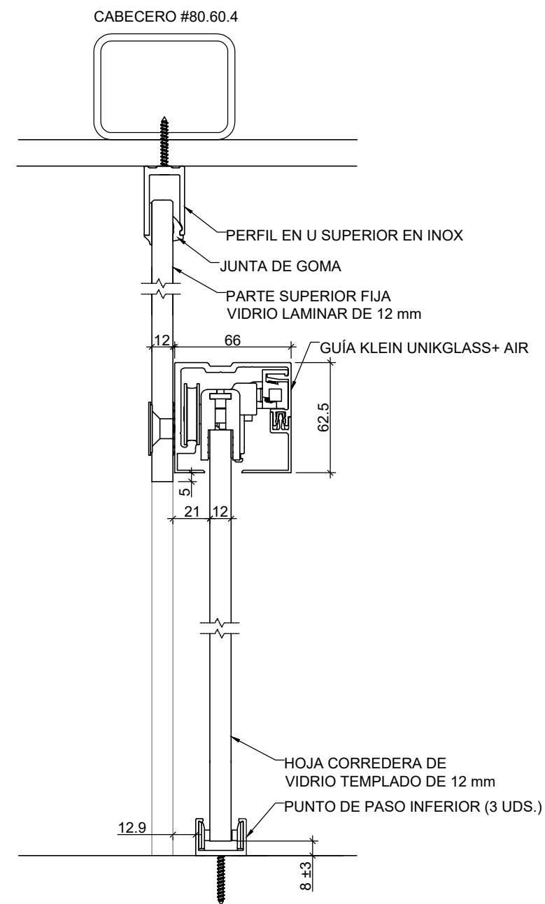
DETALLE DE SECCIÓN DE PUERTA CORREDERA
