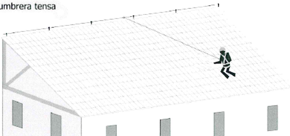
Cumbrera flexible
