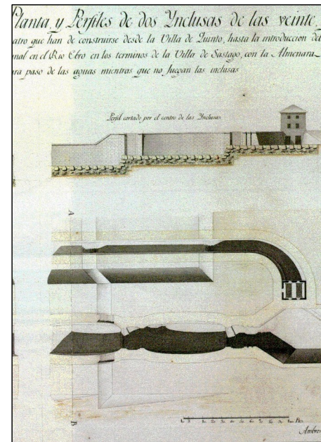
MODELO DE INCLUSA (PROYECTO ORIGINAL)
