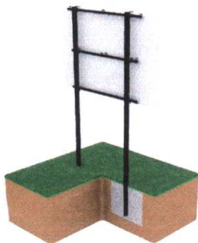
Estructura metálica (ME011L) + anclajes (PV010)
