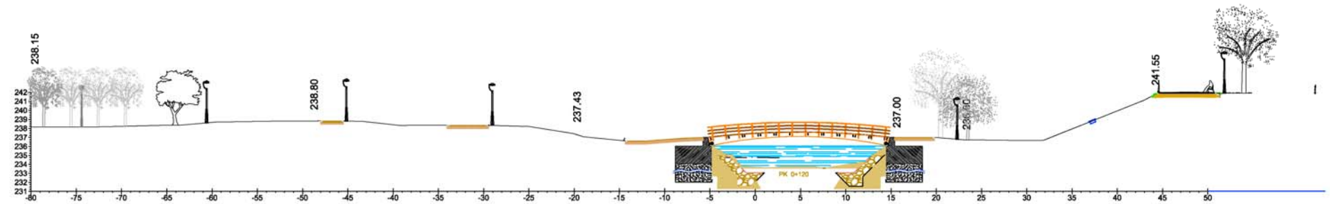
SECCIÓN 4-4'
