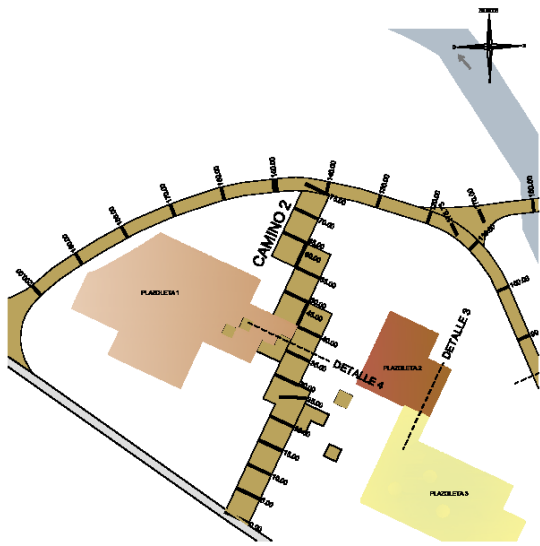
PLANTA PAVIMENTACIÓN E: 1/1.000
