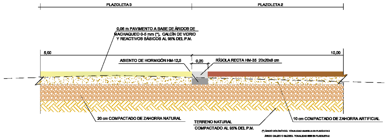
DETALLE 3. PAVIMENTACIÓN PLAZOLETA 2 Y 3 E: 1/20
