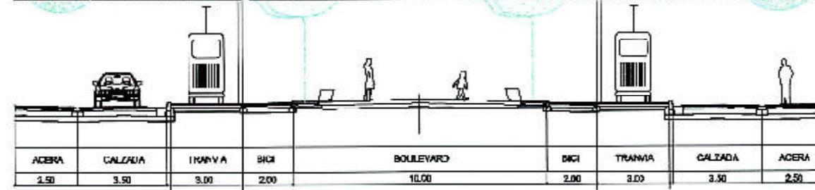
SECCION CON POSIBILIDAD DE TRANVIA
