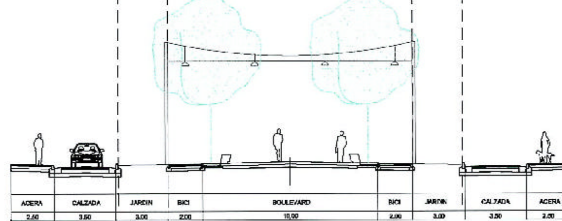
SECCION DE 32 m. BARRIO OLIVER
