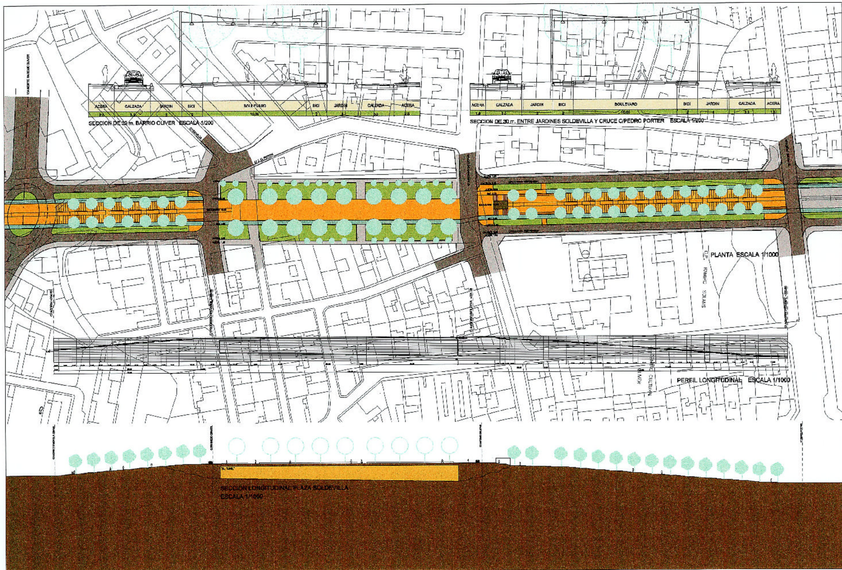
PLANTA Y SECCIONES ESCALA 1/1000 1/200 AVANCE DE ORDENACION DEL CORREDOR VERDE OLIVER-VALDEFIERRO
