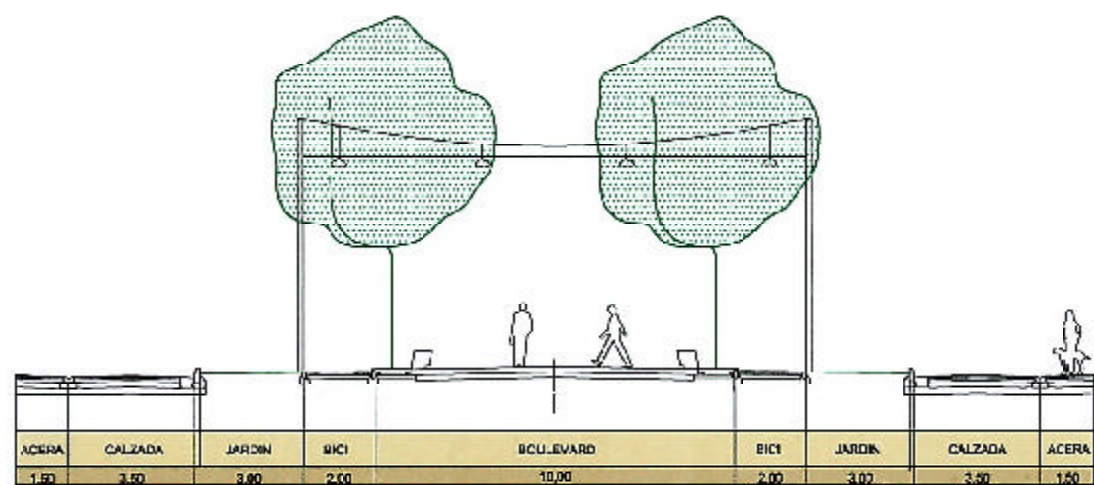
SECCION DE 30 m. ENTRE JARDINES SOLDEVILLA Y CRUCE CIPEDRO PORTER
