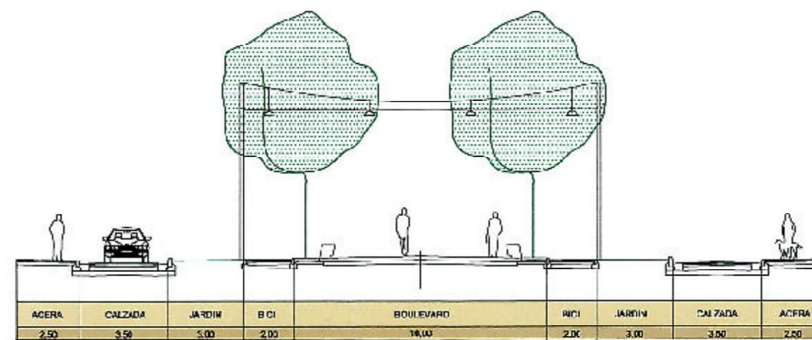
SECCION DE 32 m. BARRIO OLIVER
