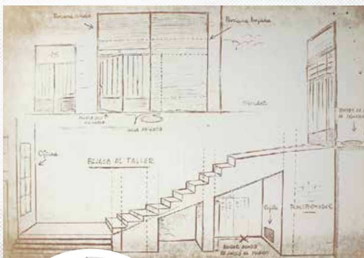
Vista exterior e interior lateral de la única puerta de entrada al taller, en dibujo de la época e infografía e imagen digitales.
